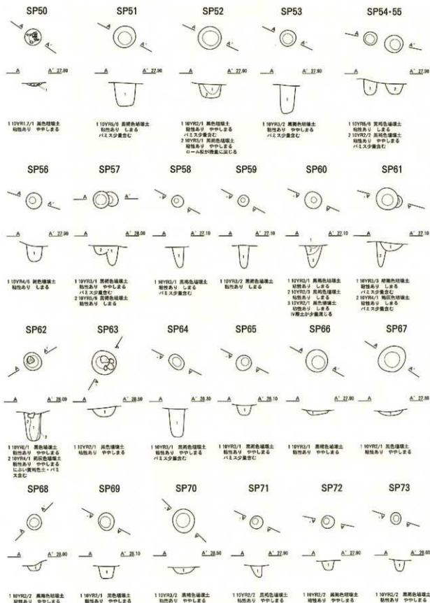
図IV-138 SP50~73平面図・断面図
