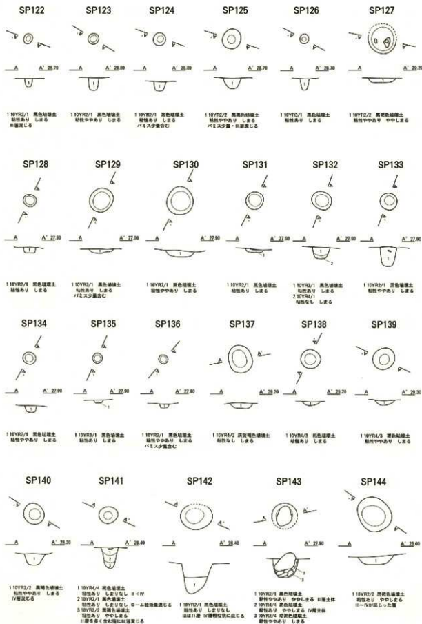
図IV-141 SP122~144平面図・断面図
