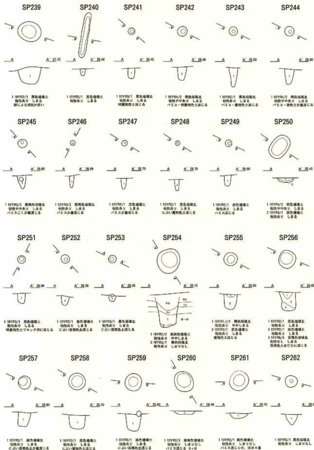
図IV-146 SP239~262平面図・断面図
