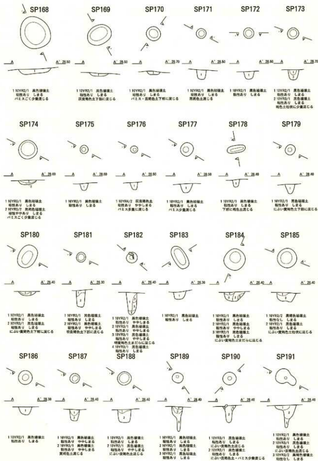
図IV-143 SP168~191平面図・断面図
