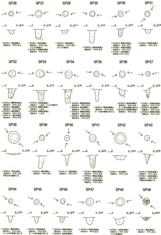
図IV-137 SP26~49平面図・断面図
