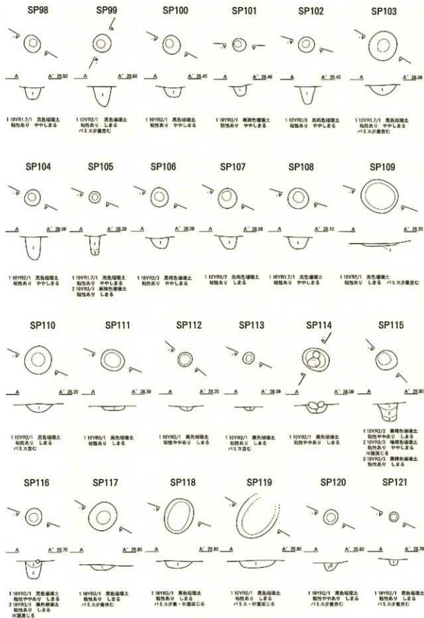
図IV-140 SP98~121平面図・断面図
