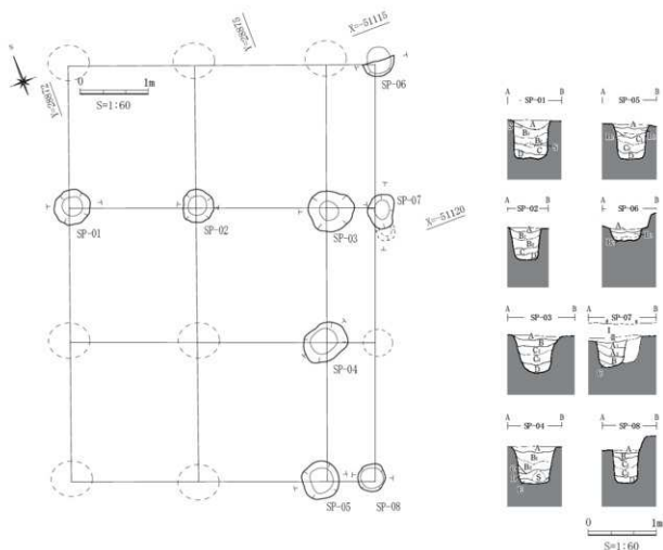
第4図 SB-01掘立柱建物跡 平面図・断面図 (1 : 60)
