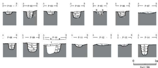
第6図 P-01～P-14 柱穴 断面図 (1:50)
