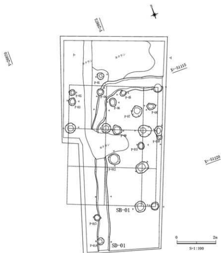
第3図 大日堂遺跡第1次調査 遺構配置図 (1:100)
