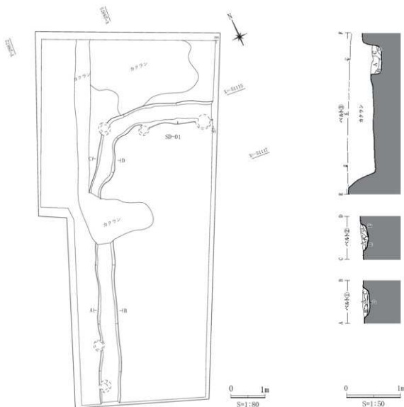
第5図 SD-01溝跡 平面図・断面図 (1:80、1:50)
