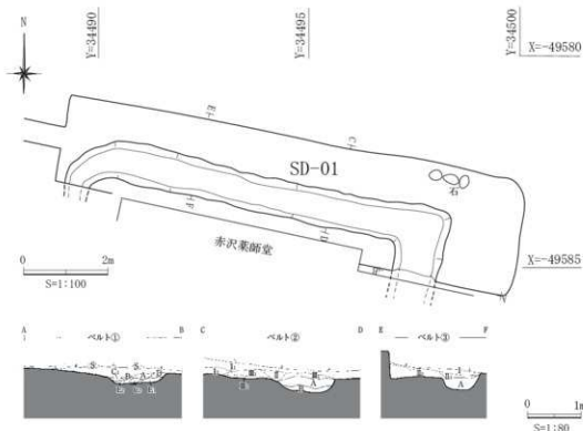
第4図 SD-01溝跡 平面図・断面図 (1:100、1:80)
