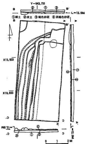
図7 試掘4 平面図
