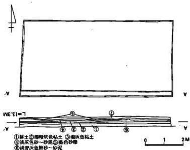
図11 試掘8 平面図
