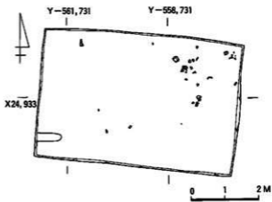
図8 試掘5 平面図
