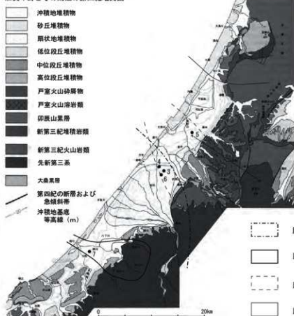
第7図 地質と土器の混和材の関係
