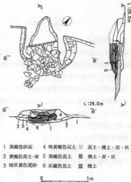
図6 2号住居址カマド
