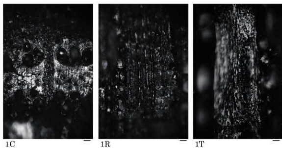
1. 試料OMH-2015-No.1 コナラ属クスギ節 C:横断面、R:放射断面、T:接線断面、スケールは0.1mm
