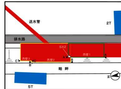
第34図 調査区西壁概略図
