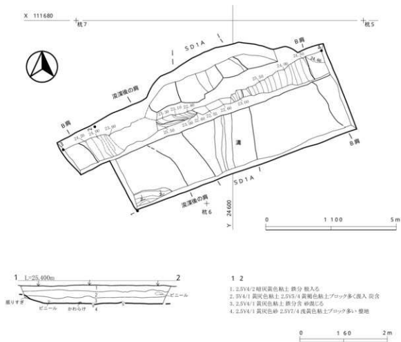
第7図 36-5 平面図
