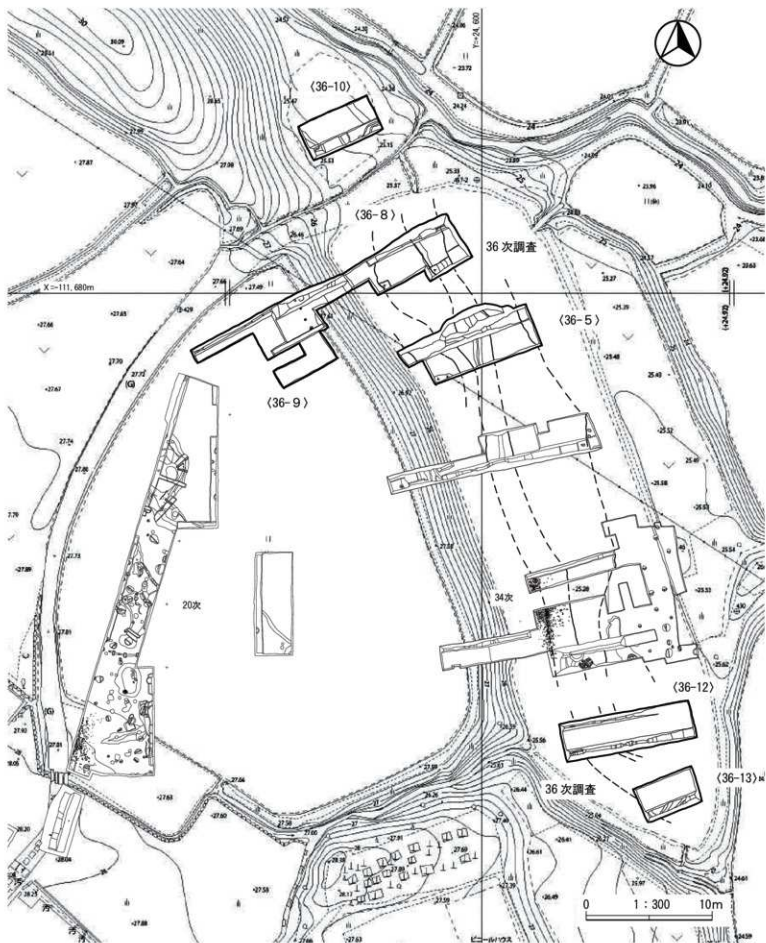
第4図 36次調査区平面図
