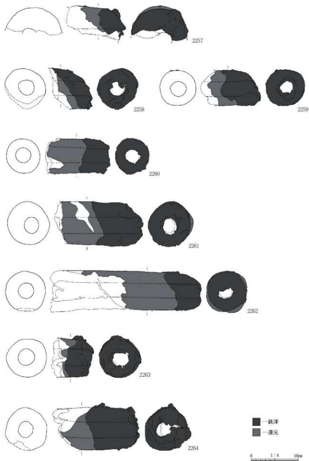
第465図 羽口 (7)
