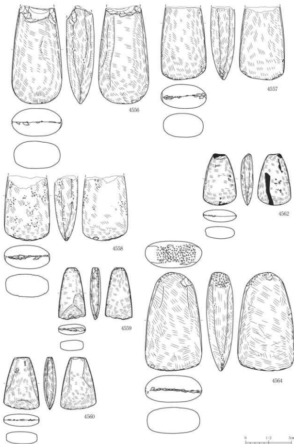
第478图 石器 (10)
