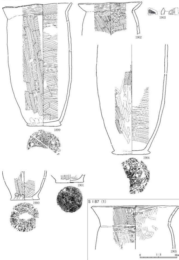
第446圖 土師器 (10)
