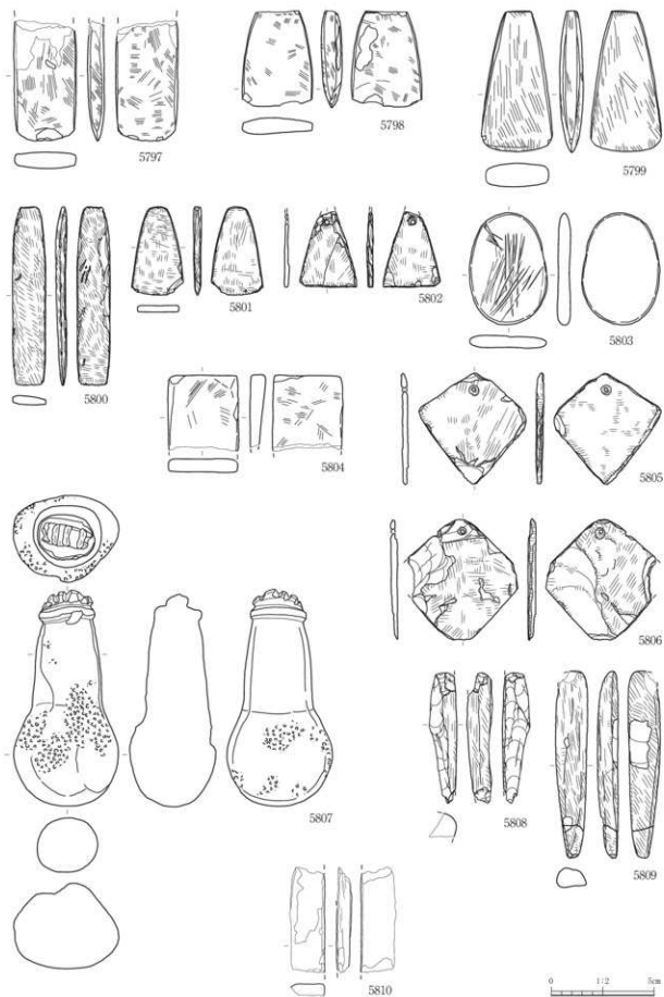
第497図 石製品 (7)
