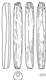
第495図 石製品 (5)
