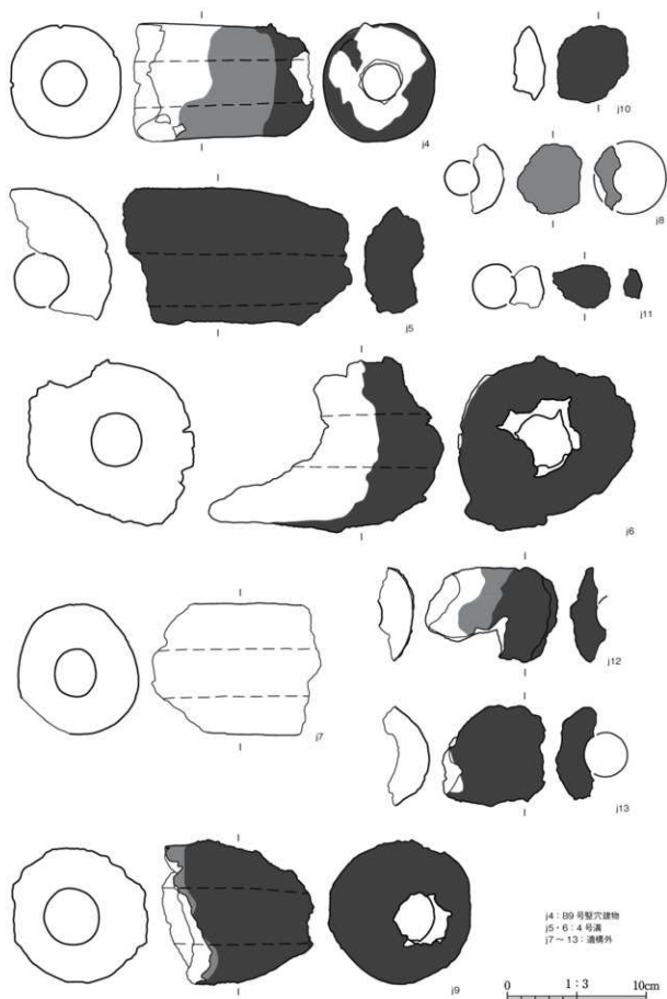
第390图 羽口(2)
