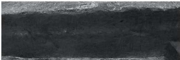
基本層序G-G'断面 (東から)
