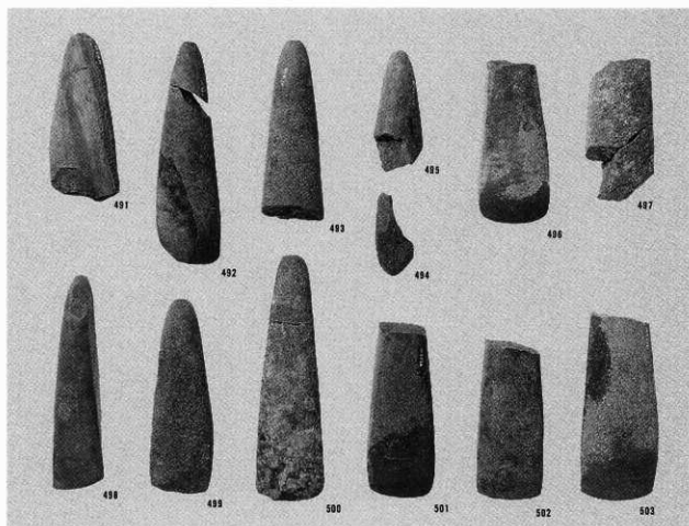
1 石斧(3) (1/3)
