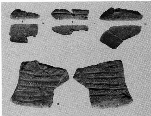
1 土偶(2) (1/2)
