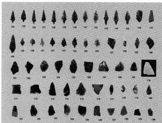
1 石鏃(3) (1/2)
