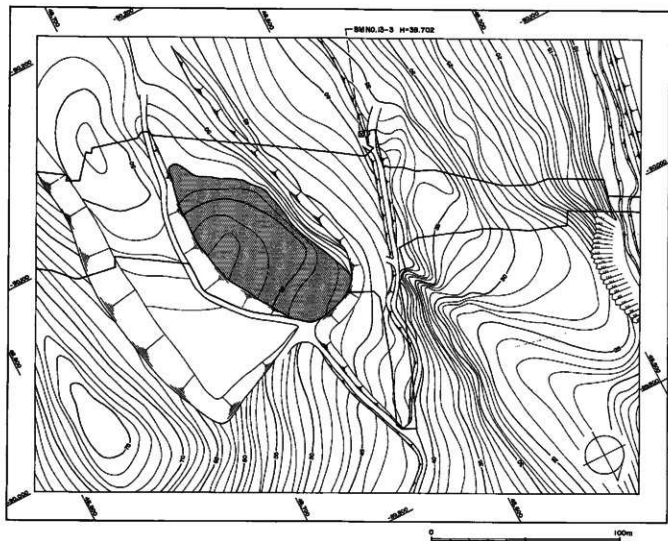
図I-2 調査区域図
