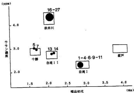
図IV-3 黒曜石片の分析結果
