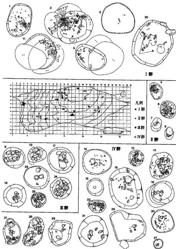
図 V-2 土壤集成図
