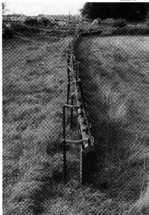
吸水管・集水管設置状況 E→W
