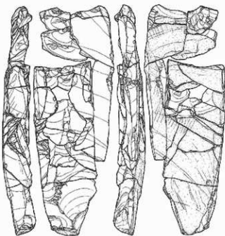
母岩26 接合64
