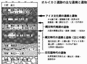
基本土層
