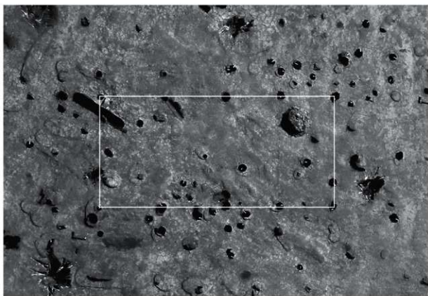
SB04 掘立柱建物跡 平面 (S→)
