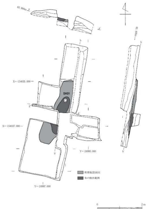
図5 第4調査区平面図・断面図 1:50
