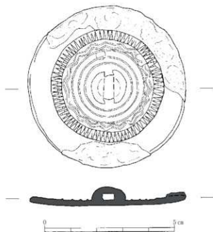
図10 重圏文鏡実測図 1 : 1
