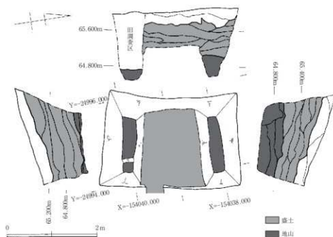
図6 第5調査区平面図・断面図 1:30
