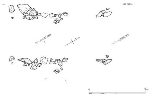
图9 第7调查区石列SX04平面图·立面图 1:30
