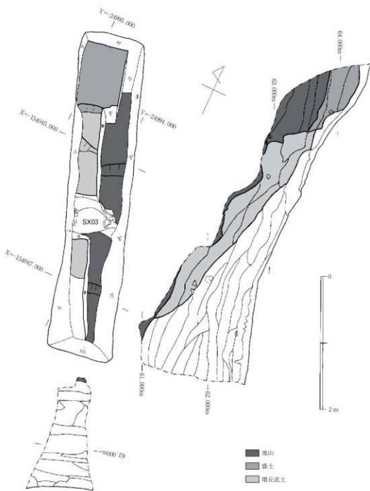
図7 第6調査区平面図・断面図 1:40
