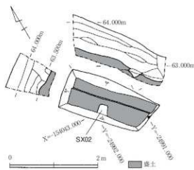
図4 第3調査区拡張区平面図・断面図 1:30
