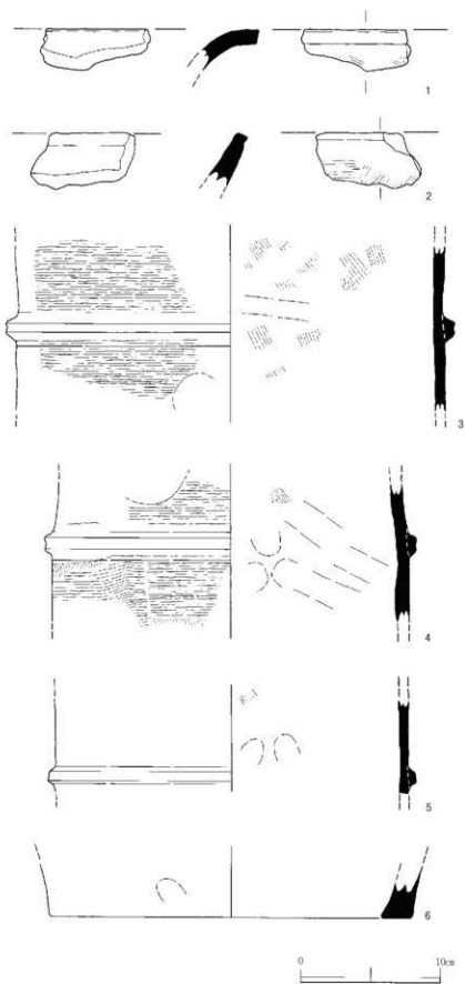
图8 凹筒埴輪实测图1 1 : 3
