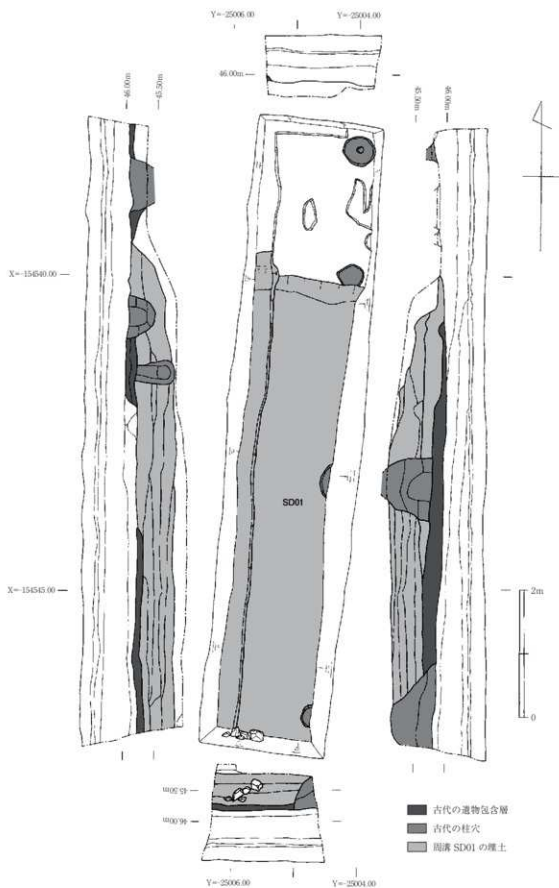
図6 第1調査区平面図・断面図 1:60
