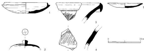
図11 土器実測図 1 : 3
