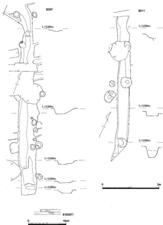
図9 SD07・11および出土遺物実測図 (S = 1/40、1/3)
