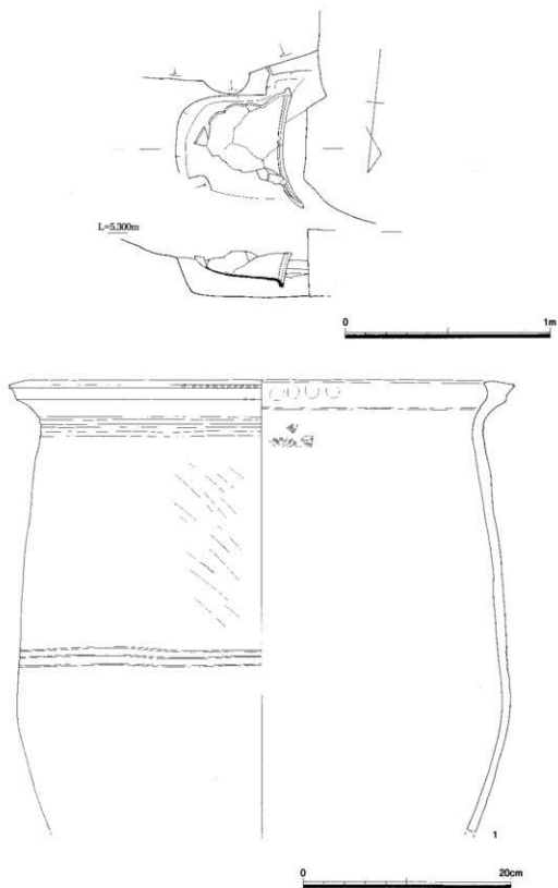
図5 ST05および出土遺物実測図 (S = 1/20、1/4)
