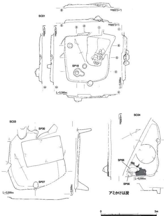
図6 SC01・03・04実測図 (S=1/60)
