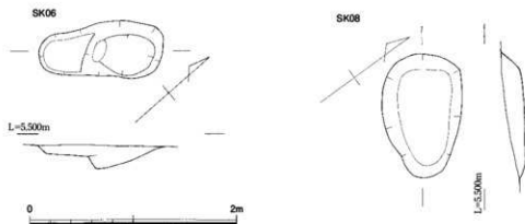
図10 SK06・08実測図 (S=1/40)
