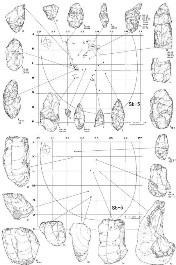
図IV-33 Sb-5の遺物(1)
