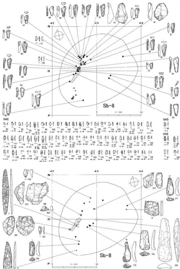
図IV-102 Sb-8の遺物(2)
