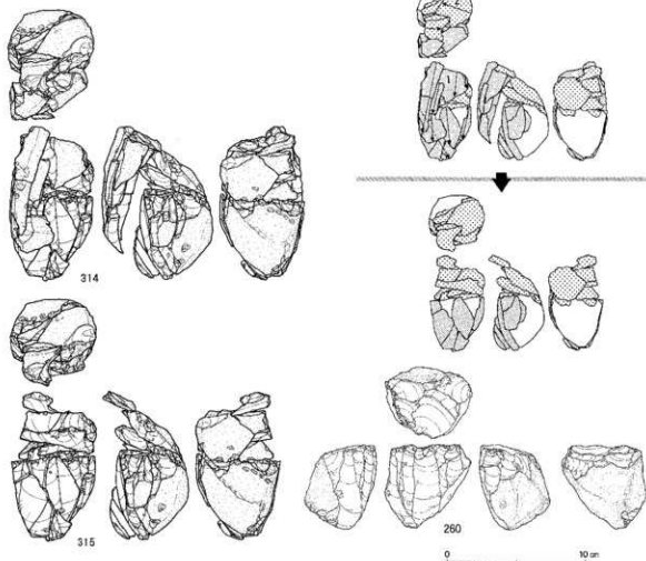
接合338分布図
