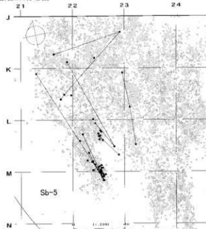
接合209分布図
