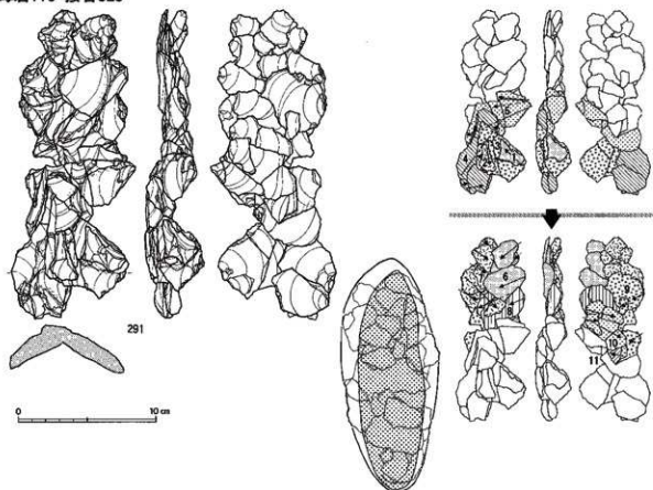
接合322分布図
