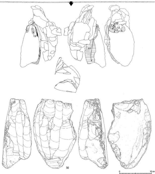
接合3244分布図
