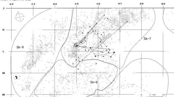
母岩113・接合318
