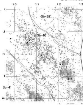
接合4266分布図
