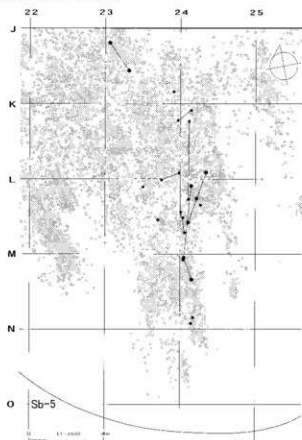
母岩61・接合44
