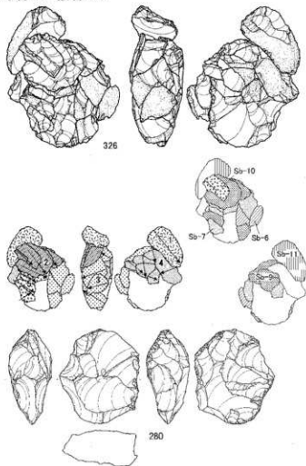
母岩147・接合470
