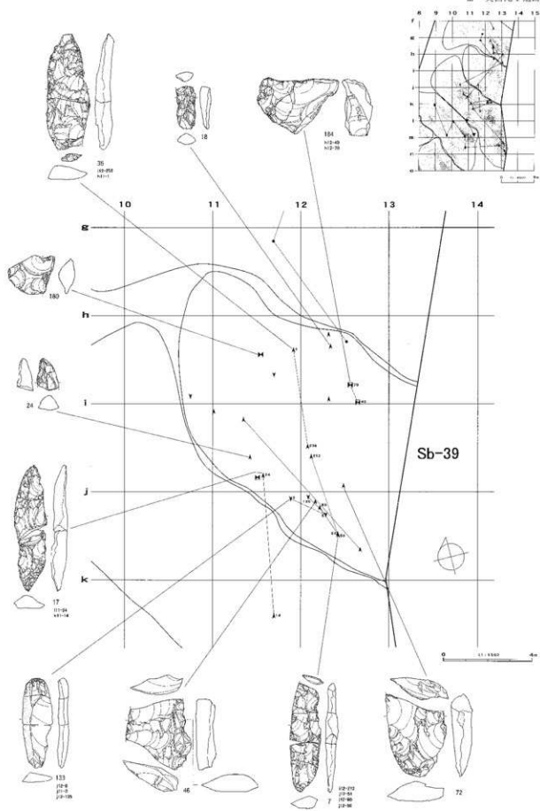
図III-383 Sb-39の遺物
