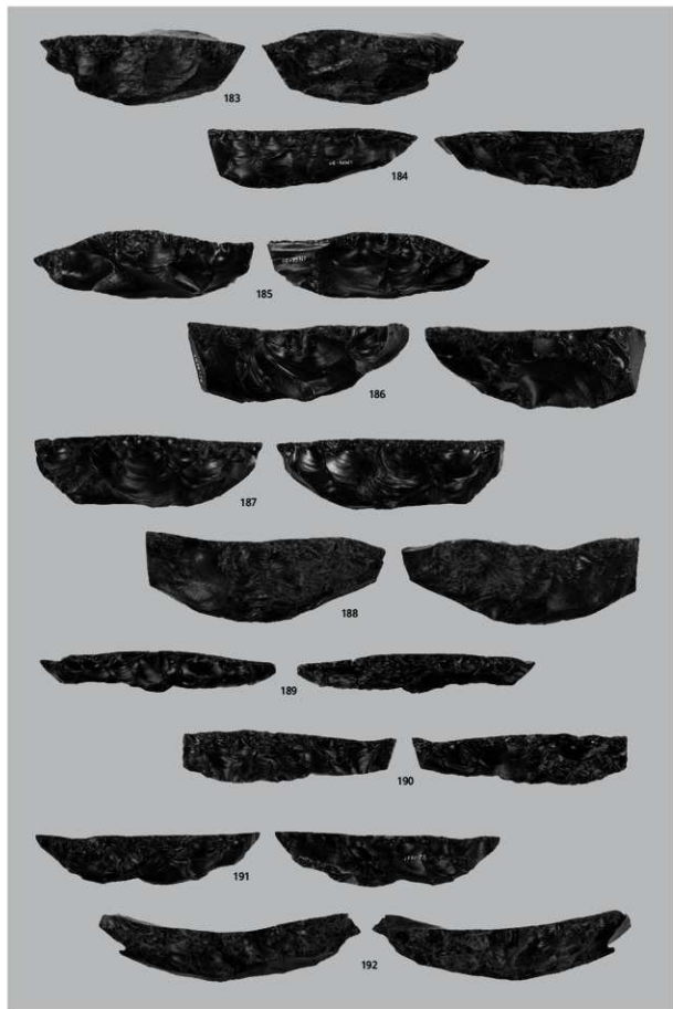
舟底形石鏡
