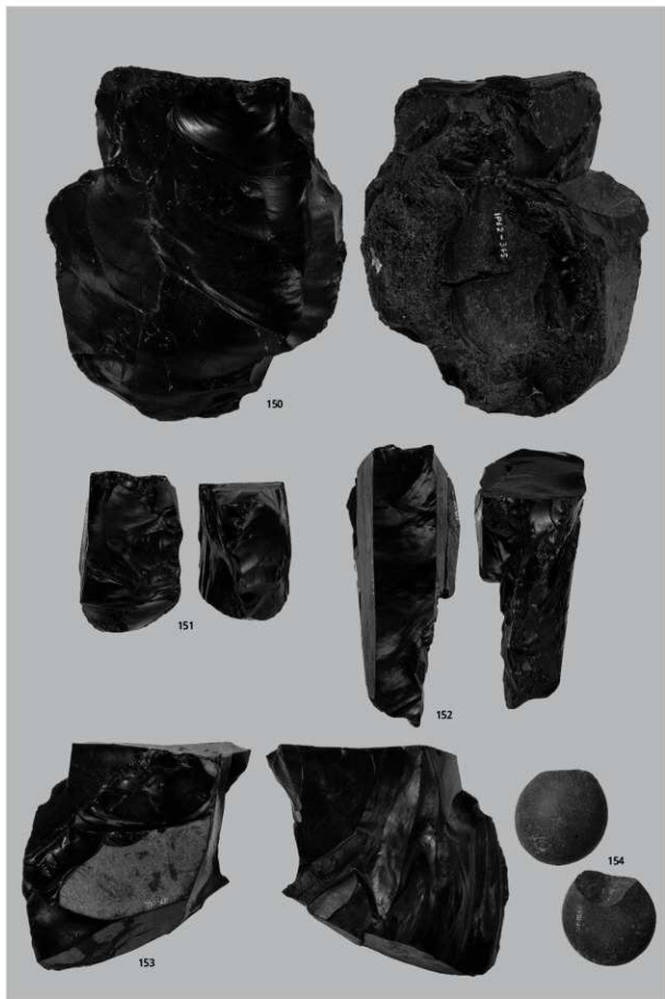
石核・敲石
