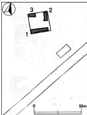
第5図 能代はまなす風力発電事業 試掘坑配置図
