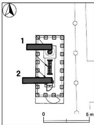
第 16 図 携帯電話無線基地局建設工事 試掘坑配置図
