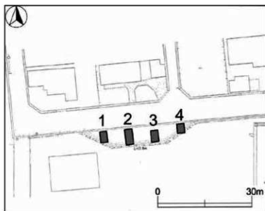
第 6 8 図 東雲中学校バス停車帯設置工事 試掘坑配置図
