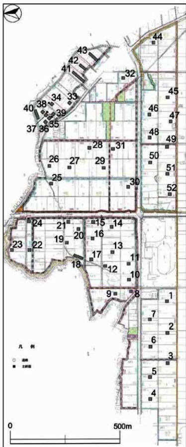
第 60 図 河戸川・浅内地区農地集積加速化基盤整備事業 試掘坑配置図
