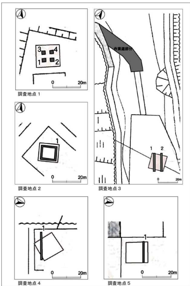
第 4 4 図 特別高圧送電線路（桧山支線）建設工事 試掘坑配置図
