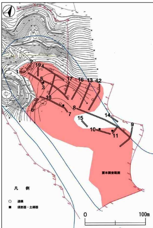
第64図 土砂採取事業 試掘坑配置図
