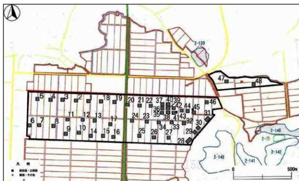
第 7 6 図 江戸川・浅内地区農地集積加速化基盤整備事業 試掘坑配置図
