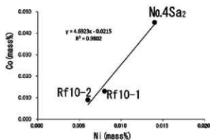
図8 調査鉄器に含まれるCu・Ni・Coの相関
