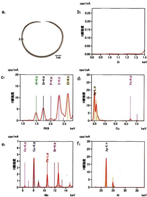
図6-1 No.7の蛍光X線分析結果(1)
