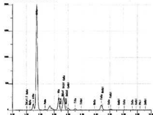
試料 No.24(a) (ⅡGP-2, 図Ⅱ-54-21)
