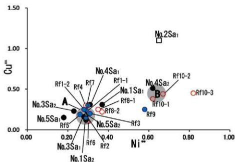
図7 調査鉄器に含まれるCu・Ni・Co三成分比
