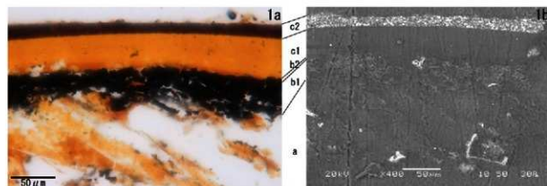
図版1 漆器椀外面赤文様部の塗膜構造 (a) と反射電子像 (b)
