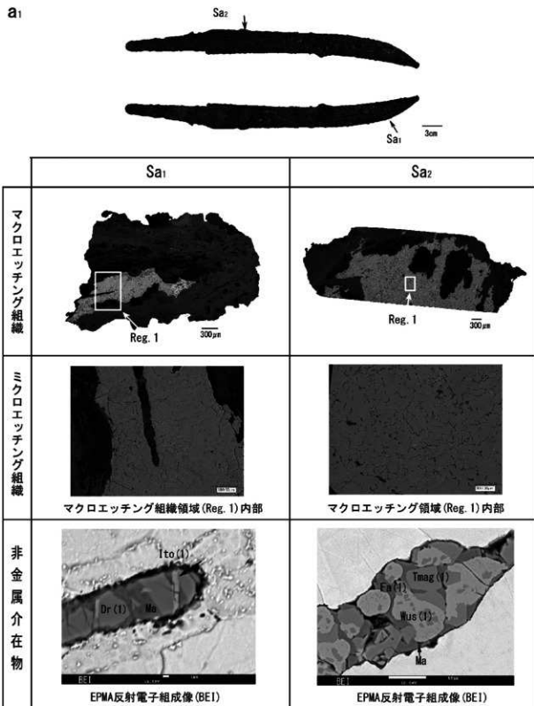
図1 No.1の組織観察結果
