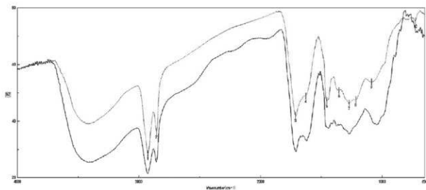
図1 漆器塗膜の赤外分光スペクトル図 (実線:塗膜試料、点線:生漆、数字:生漆の赤外吸収位置)
