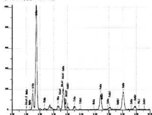
試料 No.17(c) (ⅢGP-2, 図Ⅲ-54-14)
