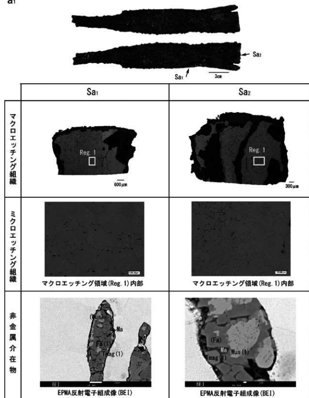
図3 No.3の組織観察結果
