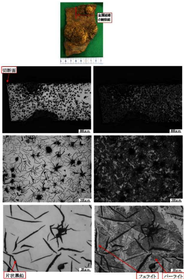
図版2 鋳（上3-9）断面の金属組織
