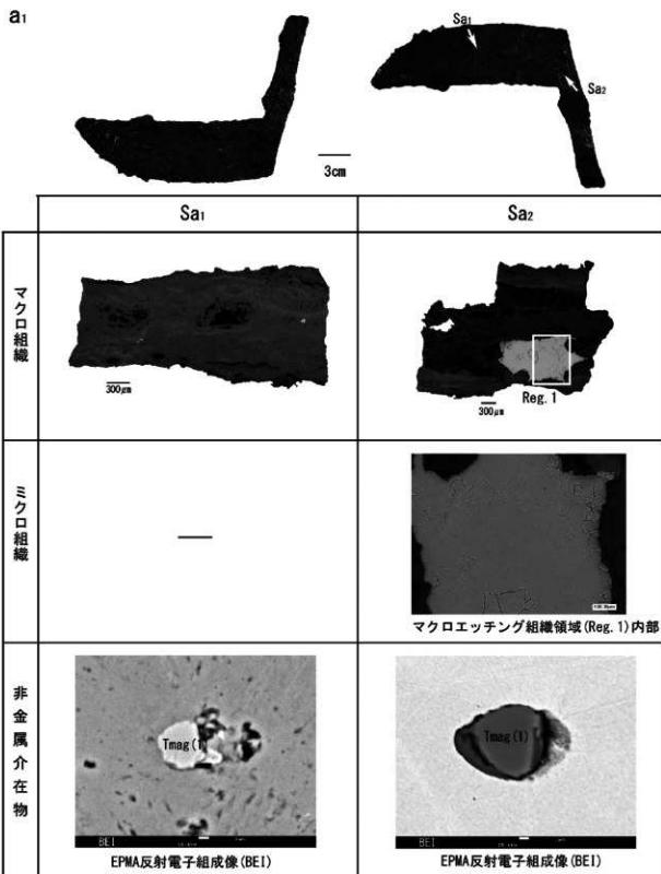
図4 No.4の組織観察結果
