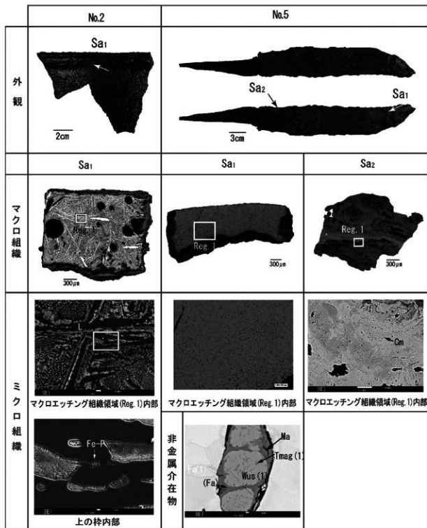
図2 No.2・No.5の組織観察結果
