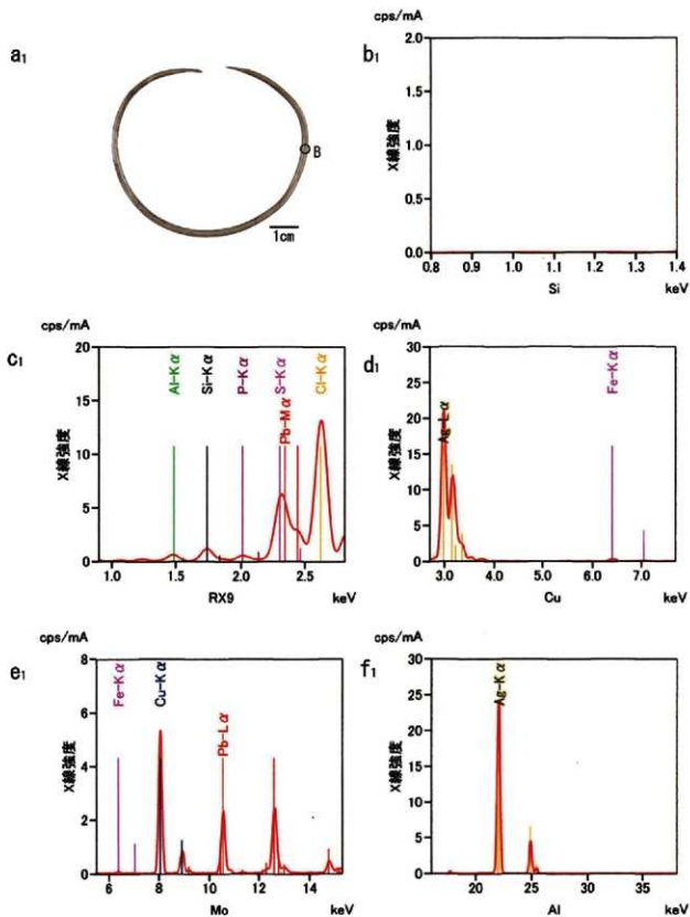
図6-2 No.7の蛍光X線分析結果(2)
