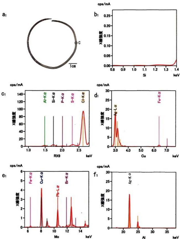
図5-3 No.6の蛍光X線分析結果（3）
