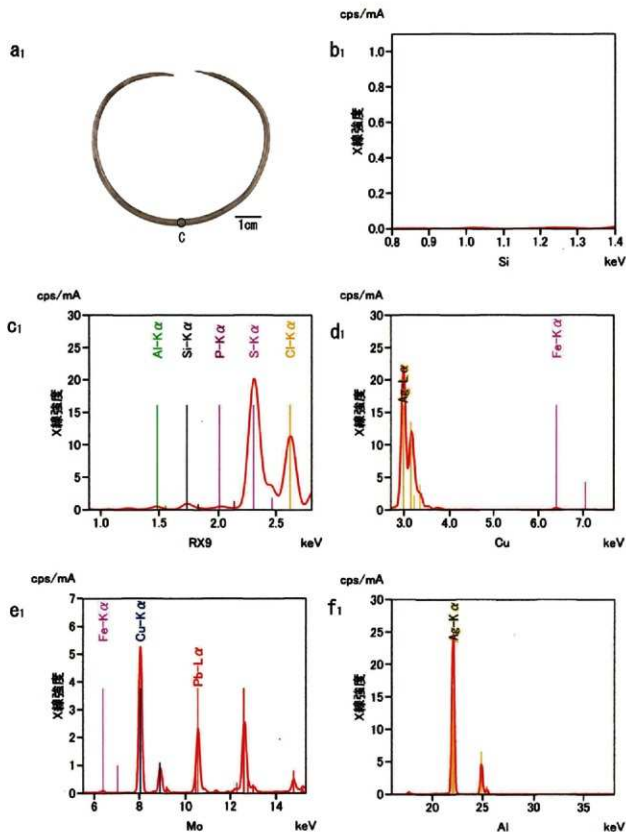
図6-3 Na7の蛍光X線分析結果(3)
