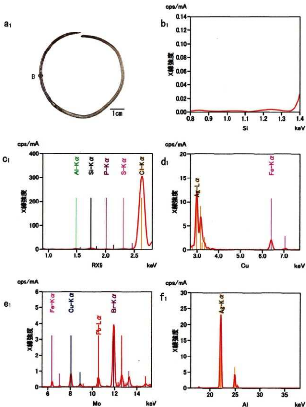
図5-2 No.6の蛍光X線分析結果(2)
