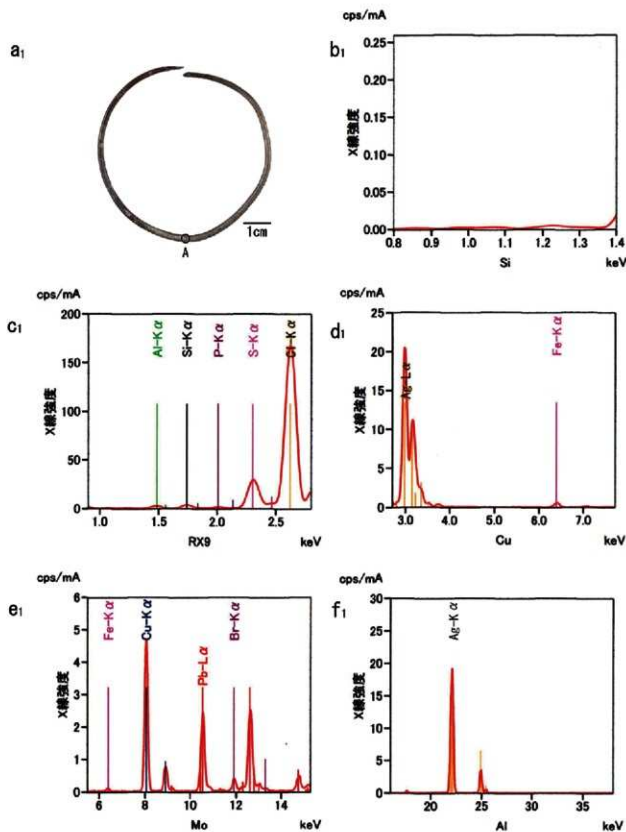
図5-1 No.6の蛍光X線分析結果(1)
