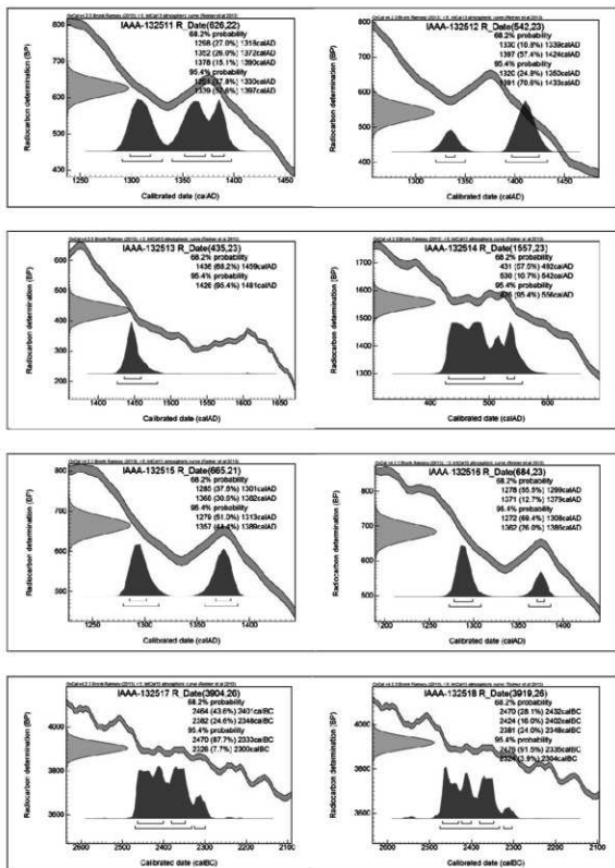
図1-2 暦年較正年代グラフ (2)
