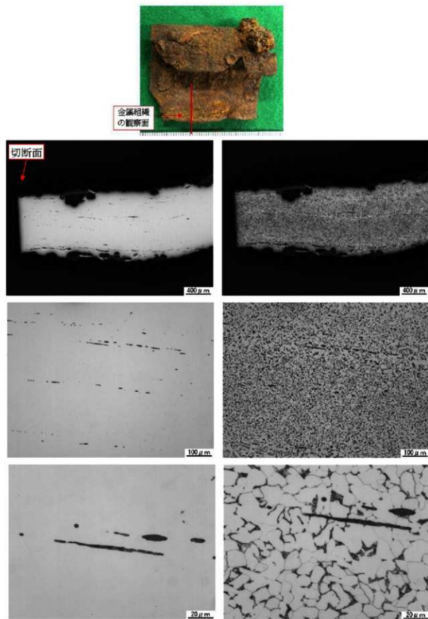
図版3 刀装具（上3-27）断面の金属組織
