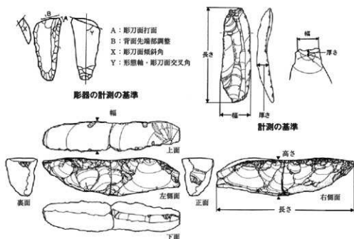
舟底形石器・細石刃核・総石刃核削片の面の呼称と計測の基準
