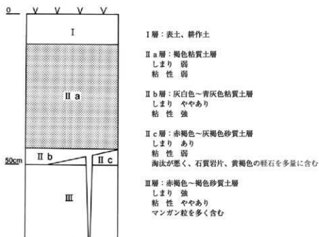
図 1-14 基本土層図
