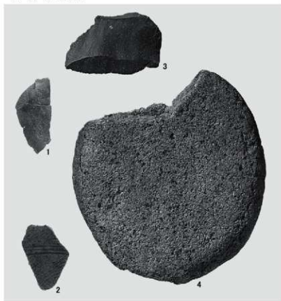
CP-41-4はS=1/3
