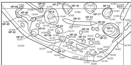
HF-1 周辺詳細図 (1/20)
