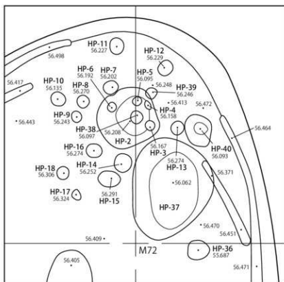
HP-2 周辺詳細図 (1/20)
