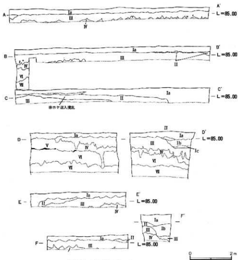
第18図 金剛寺原第2遺跡の土層図
