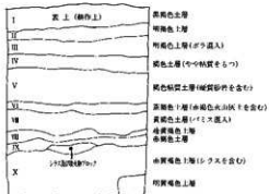
第3図 金剛寺原第1遺跡土層断面図
