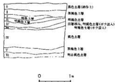
14-C 南壁セクション
