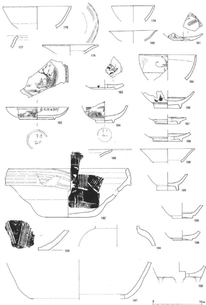
Fig. 35 C-I区SC51出土遺物実測図(1)
