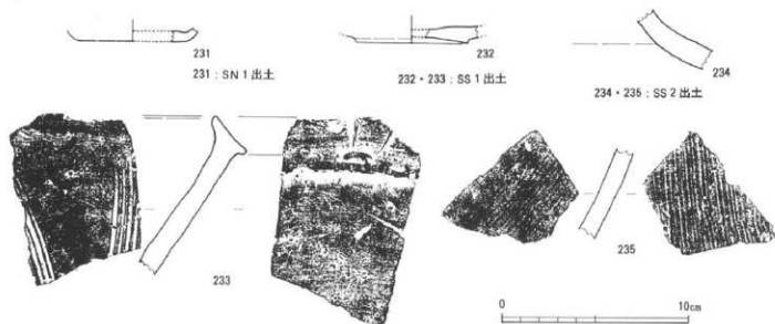
Fig. 40 その他の遺構出土遺物実測図
