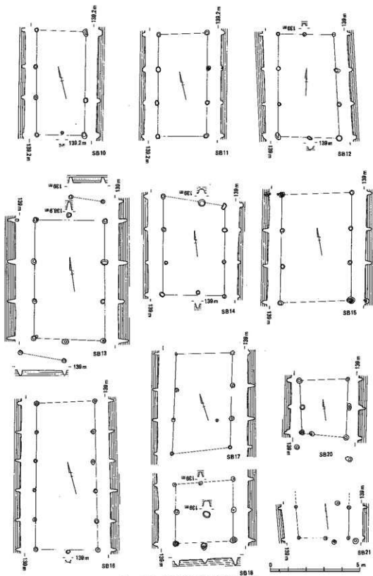
Fig. 27 掘立柱建物実測図 (2)
