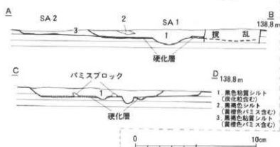
Fig. 32 土坑および竪穴状遺構実測図
