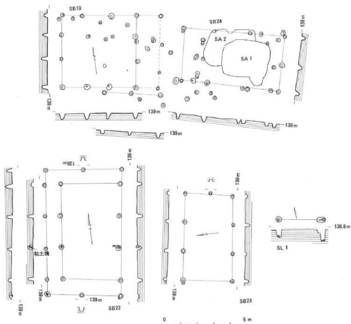
Fig. 28 掘立柱建物実測図 (3)
