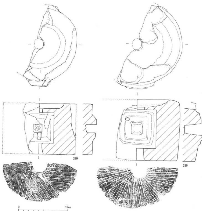
Fig. 38 C-I区SC51出土遺物実測図（4）
