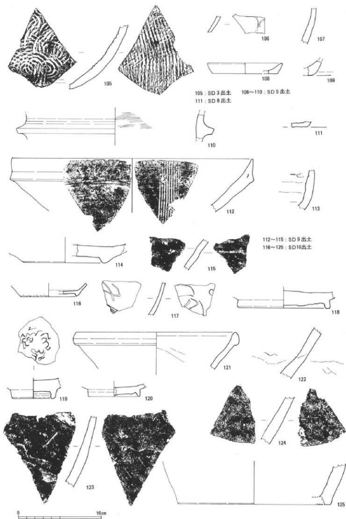
Fig. 16 A区沟状遗构出土文物实测图 (2)
