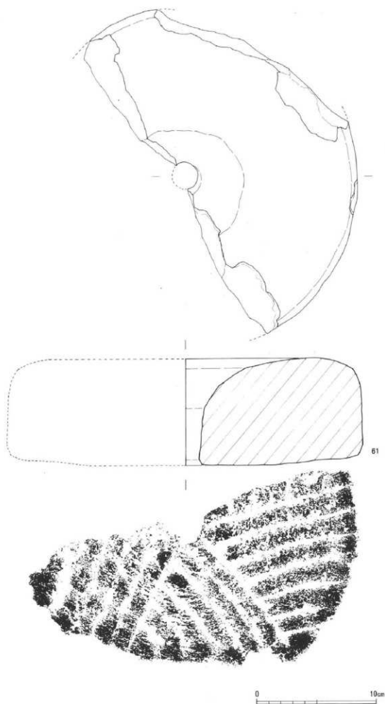
Fig. 7 歴史時代の遺物実測図 (2)
