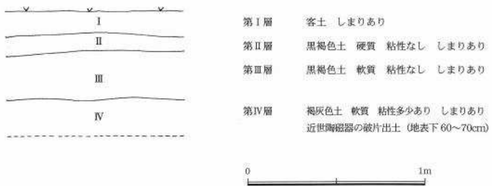
第10図 大手地区個人住宅建設予定地土層断面図(S=1/20)
