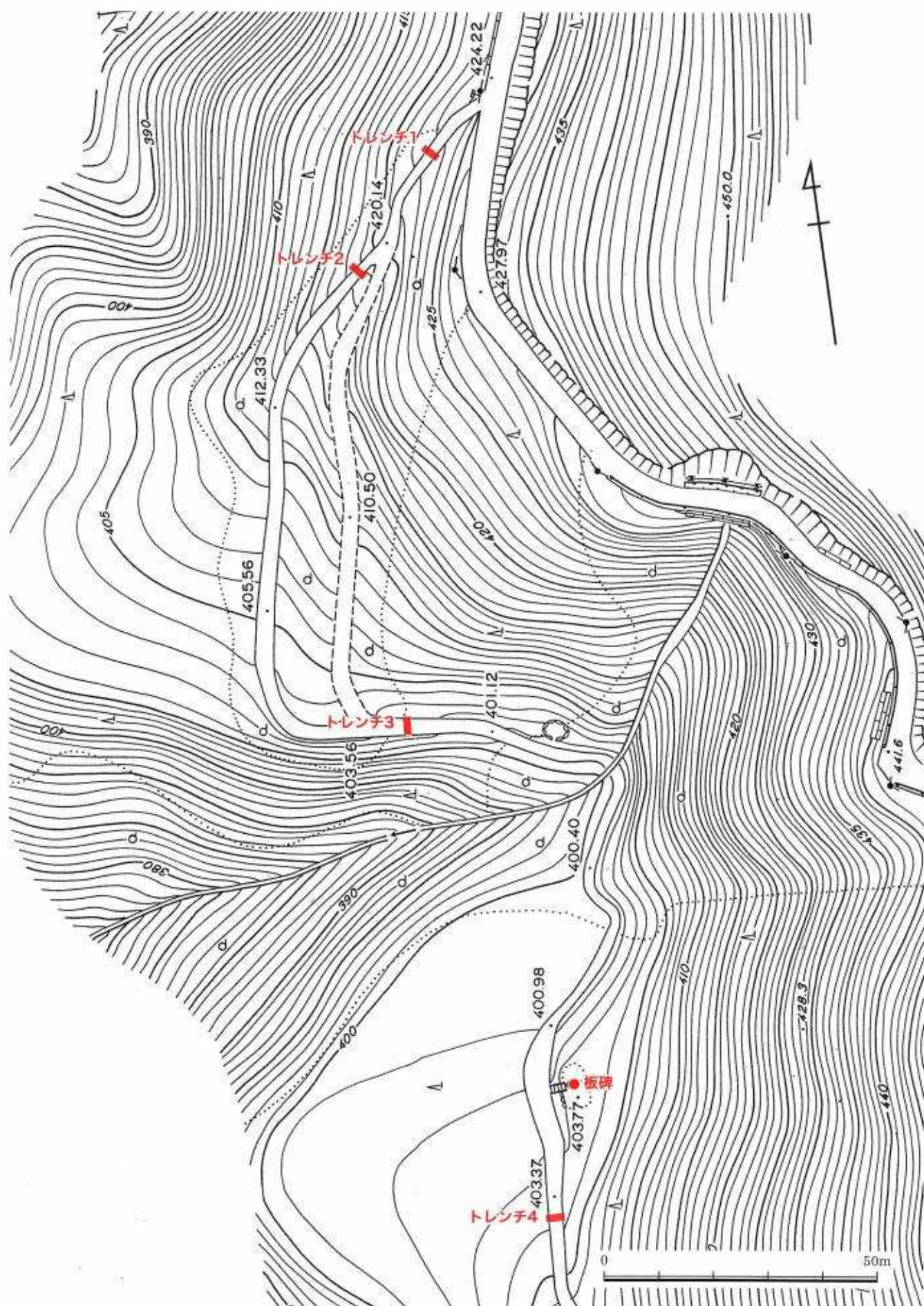
第12図 平成24年度分取造林伐採搬出予定地トレンチ配置図(S=1/1,000)
