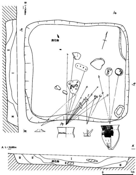
第9圖 竪穴式住居跡 (SA-1) 実測圖
