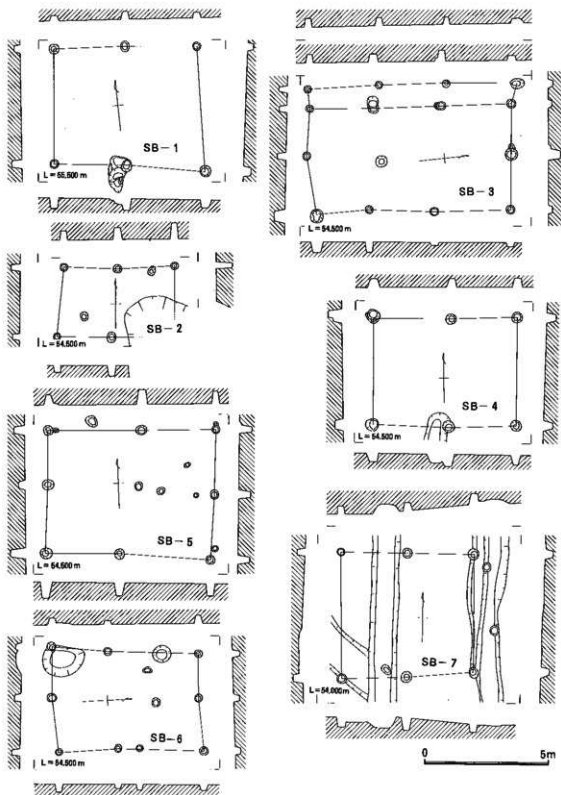
第11圖 掘立柱建物跡実測図
