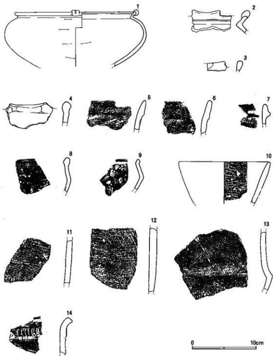
第5圖 縄文土器実測圖
