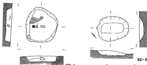
第22図 遺構実測図
