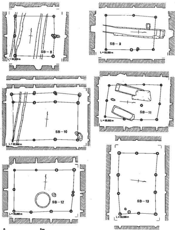
第12图 掘立柱建物跡実測图
