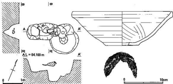
第13図 SC-1 及び出土遺物実測図
