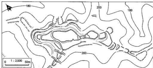
第2図 三俣城縄張り図（千田嘉博原図作成 山之口町教育委員会提供） 『宮崎県中近世城館跡緊急分布調査報告書Ⅱ』（1993 宮崎県教育委員会）より転載
