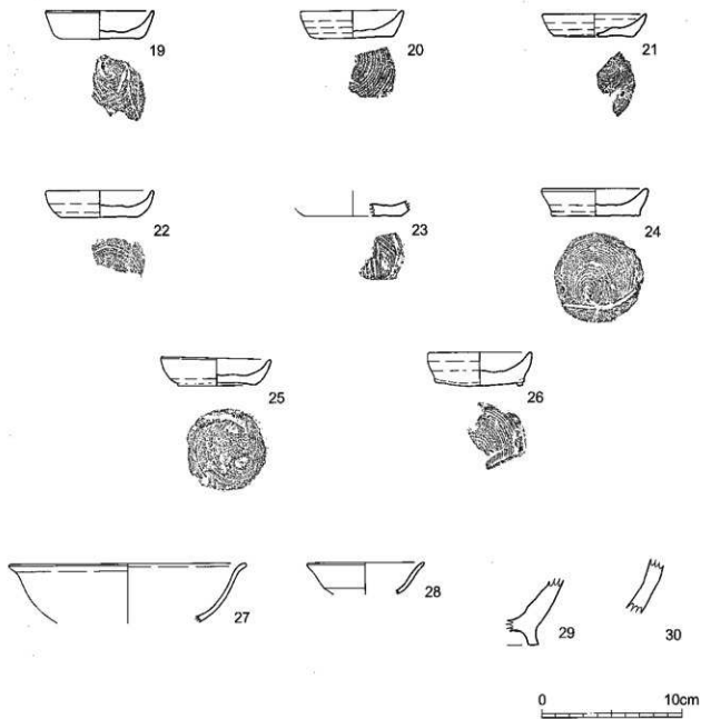
第9圖 遺物実測図2 (土師器・磁器 S=1:3)
