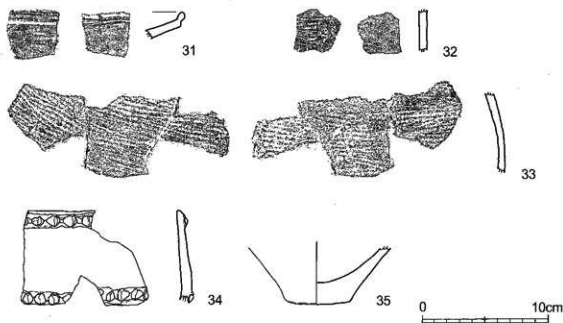
第10図 遺物実測図3 (縄文土器 S=1:3)
