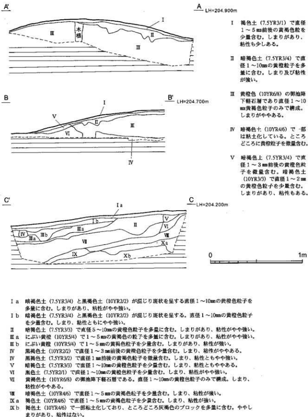
第7図 土層断面図1 (S=1:20)
