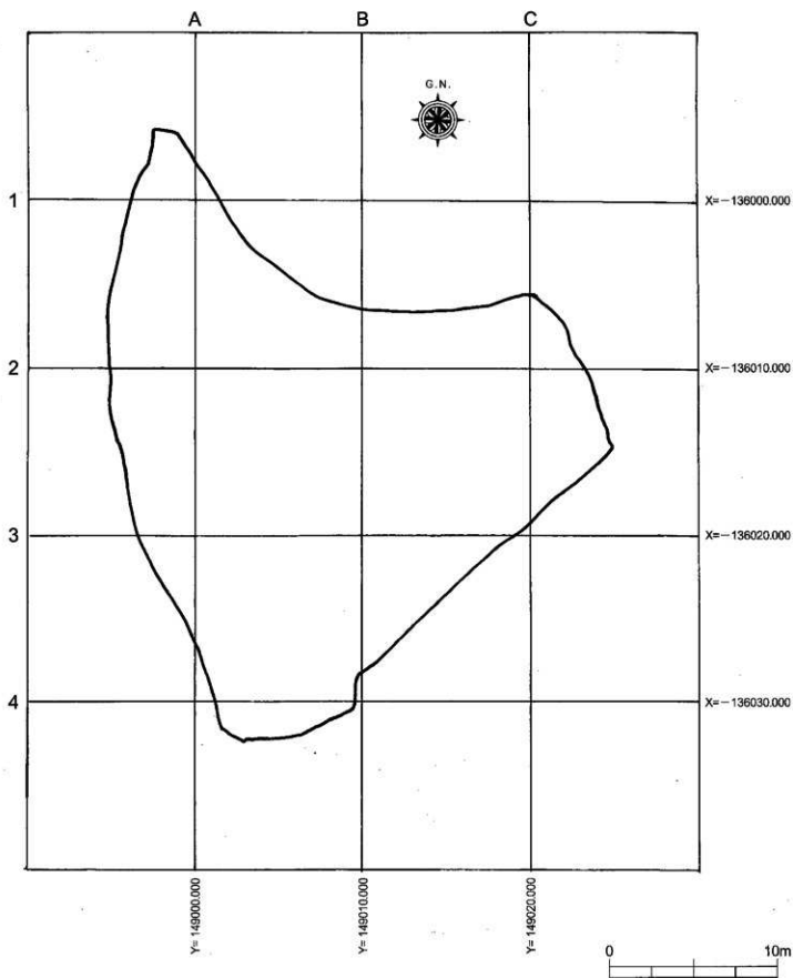
第4図 グリッド配置図 (S = 1 : 250)
