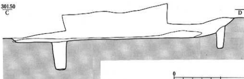
第14图 7号住居実測図
