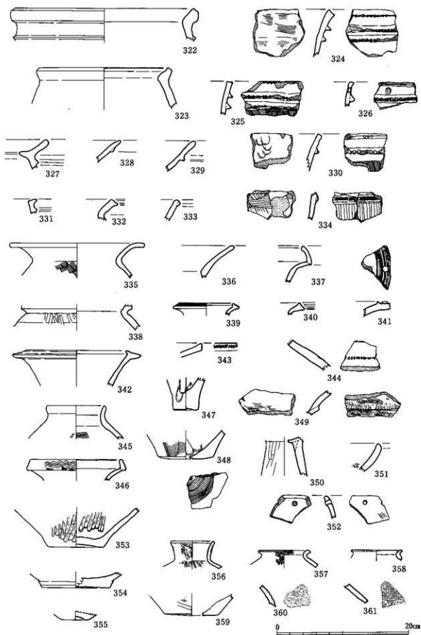
第43图 濠沟外出土遗物实测图(1)
