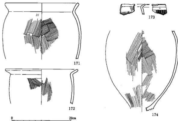
第22図 11号住居出土遺物実測図
