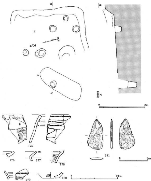
第23図 12号住居および出土遺物実測図
