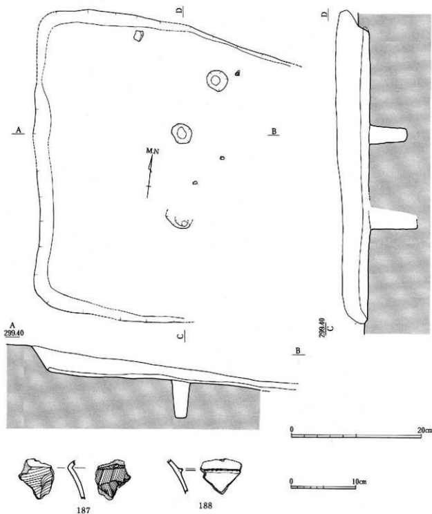
第26図 15号住居および出土遺物実測図
