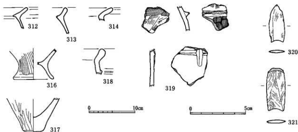
第42図 25号住居出土遺物実測図
