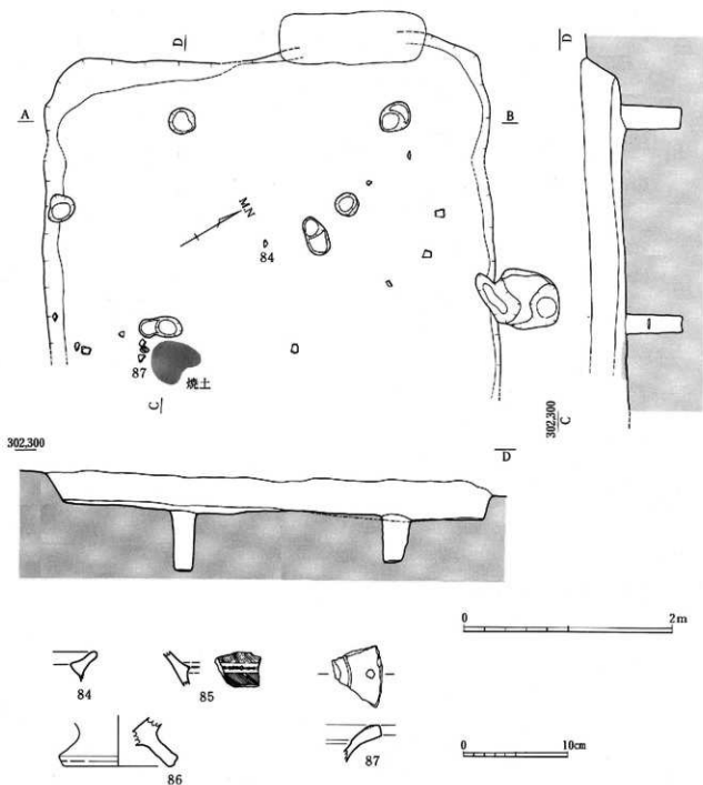
第9図 2号住居および出土遺物実測図
