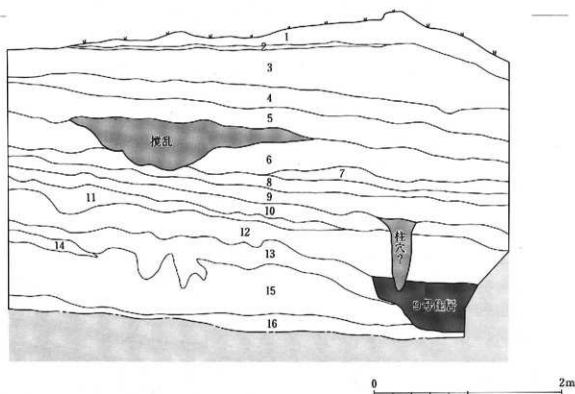
第2図 土層図
