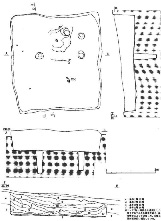
第 33 図 19号住居実測図
