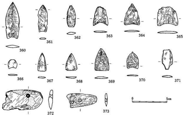
第44図 遺構外出土遺物実測図(2)
