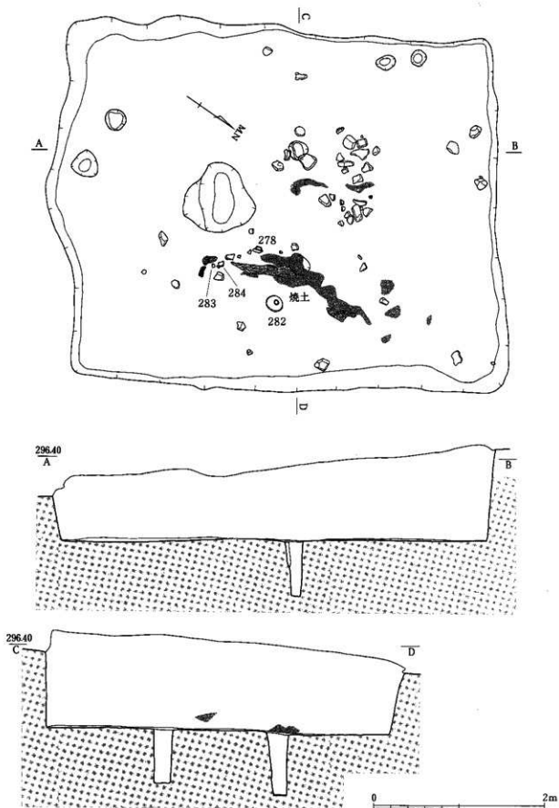
第36图 21号住居实测图
