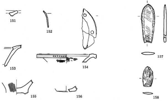
第18図 9号住居および出土遺物実測図
