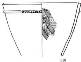
第13図 6号住居および出土遺物実測図
