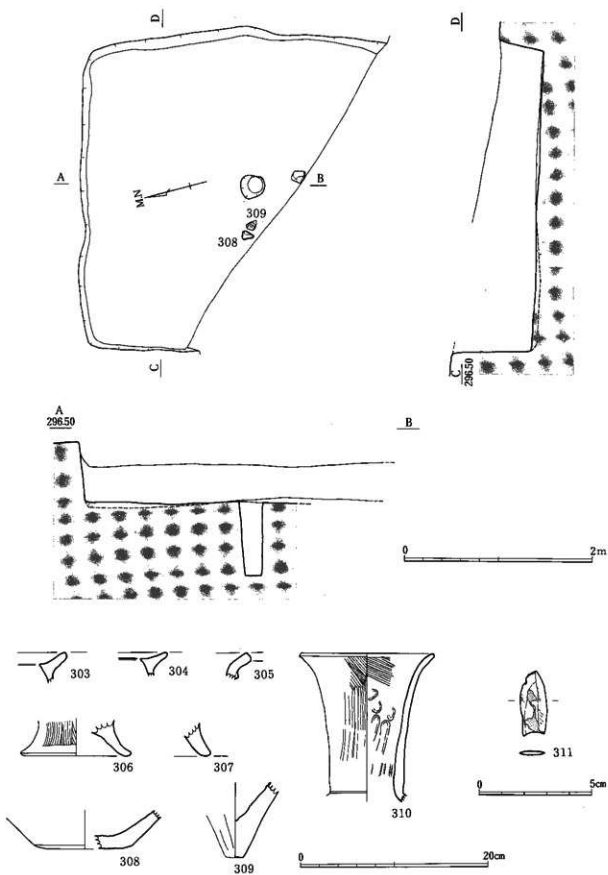
第40図 24号住居および出土遺物実測図
