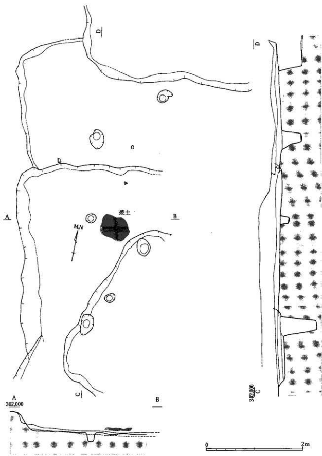
第10图 3·5号住居实测图
