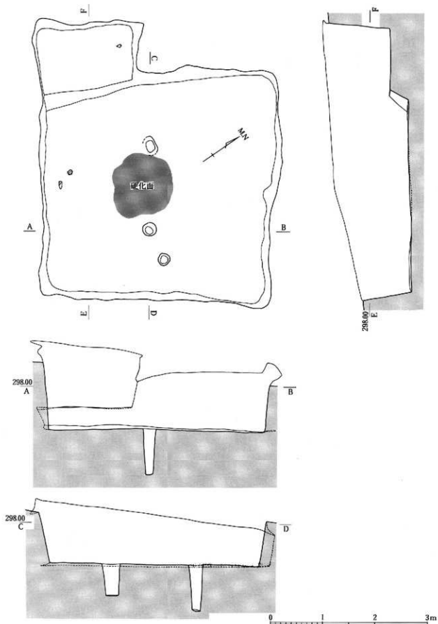
第28图 17号住居实测图
