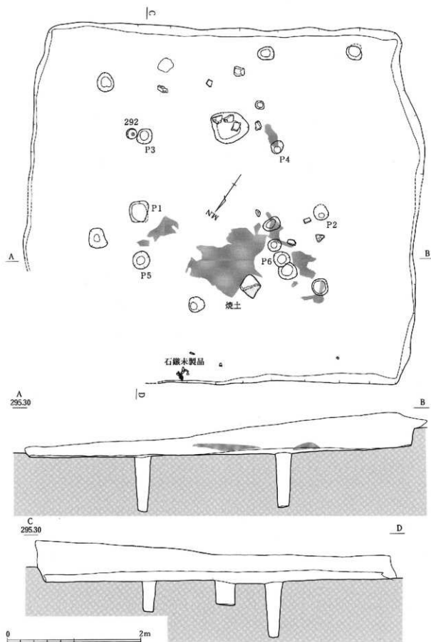
第37图 22号住居実測図
