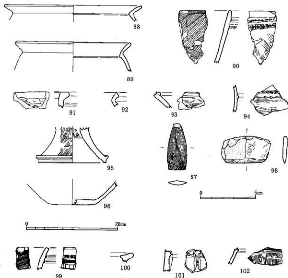
第11図 3・5号住居出土遺物実測図
