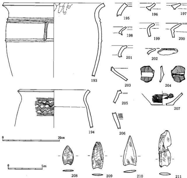
第29図 17号住居出土遺物実測図
