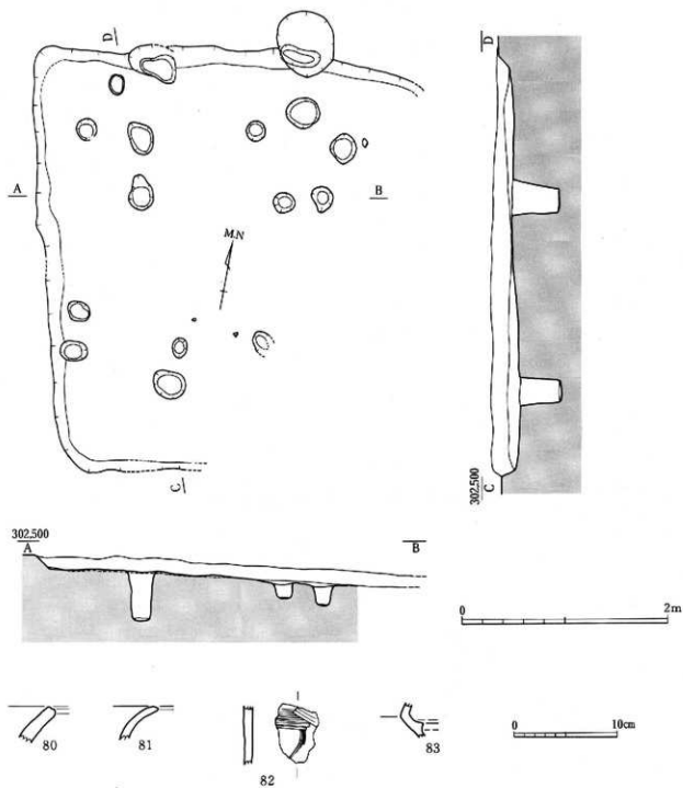
第8図 1号住居および出土遺物実測図
