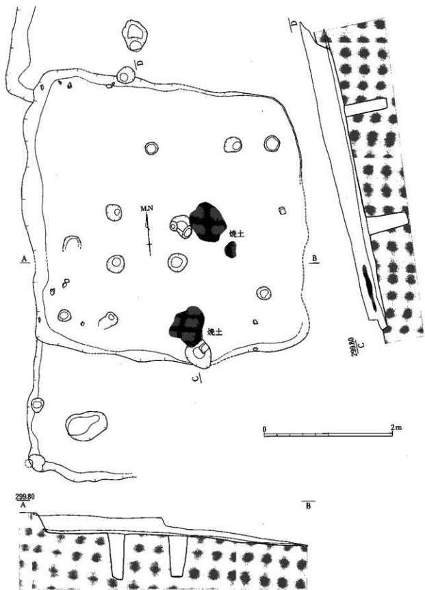
第 21 图 11 号住居实测图
