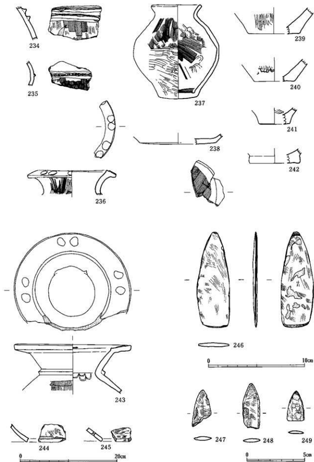
第32图 18号住居出土遺物実測図(2)
