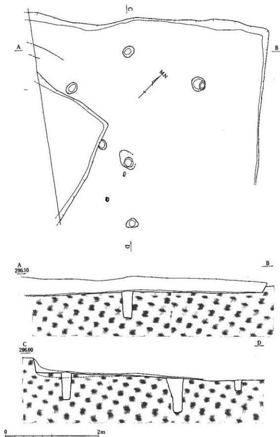
第41图 25·26号住居夹测图
