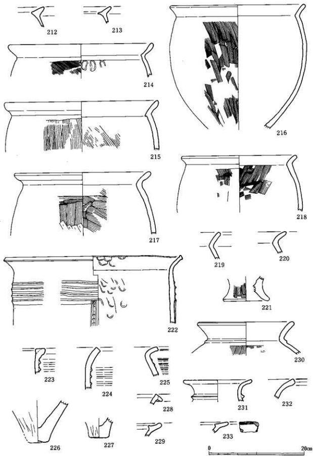
第31图 18号住居出土遗物实测图(1)
