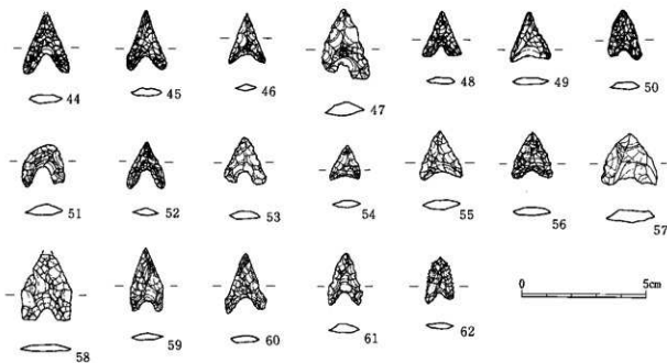
第6図 石器実測図(1)
