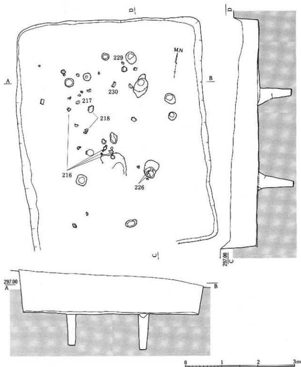
第30図 18号住居実測図
