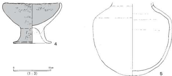
第30図 7T 出土遺物実測図 (S=1/3)
