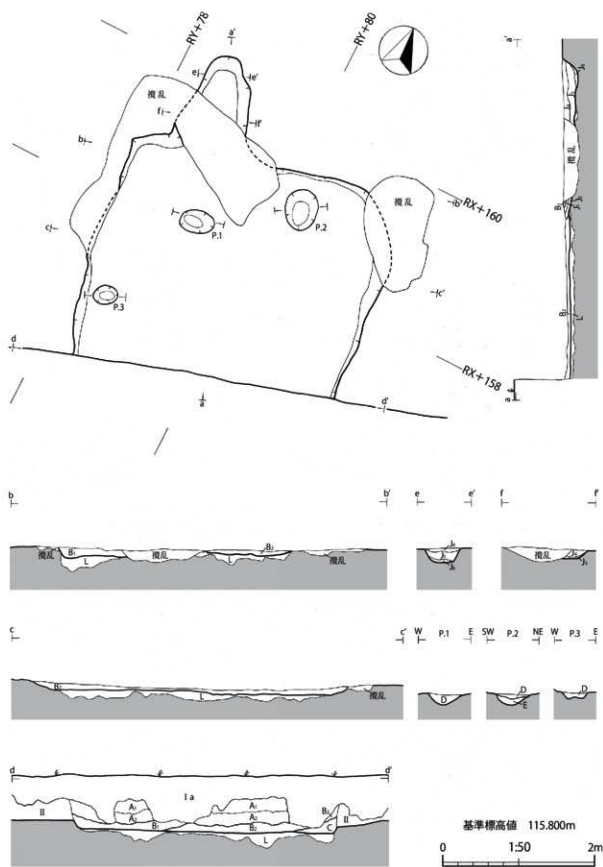
第 8 图 RA 058 竖穴建物跡
