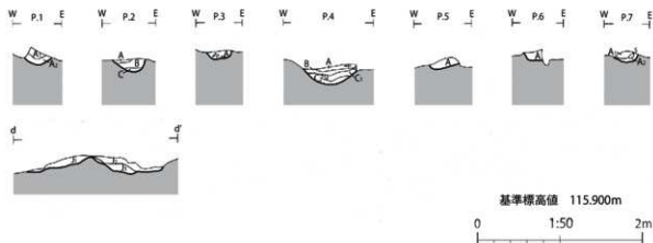
第 11 図 RA 059 竪穴建物跡 (2)
