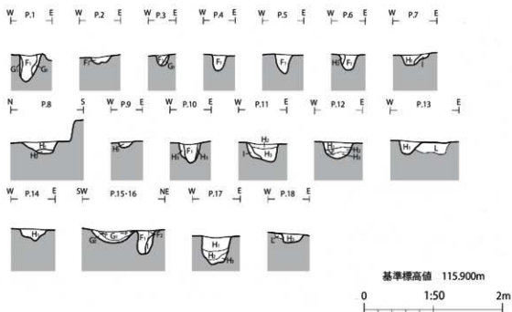
第6図 RA 057 竪穴建物跡(2)
