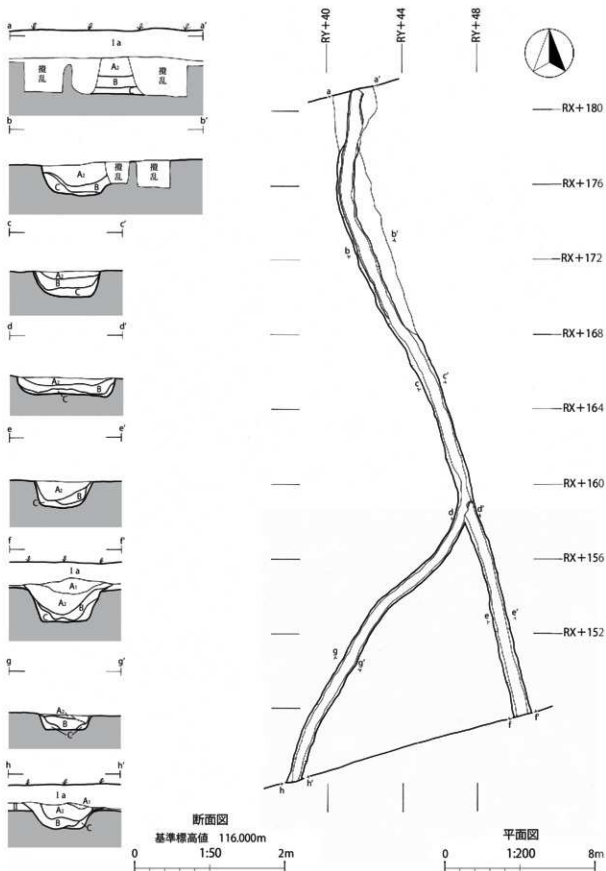
第 15 図 RG 012 溝跡
