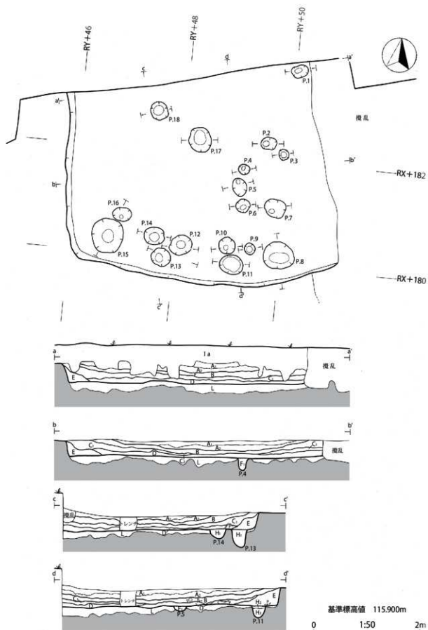
第5図 RA 057 竪穴建物跡(1)
