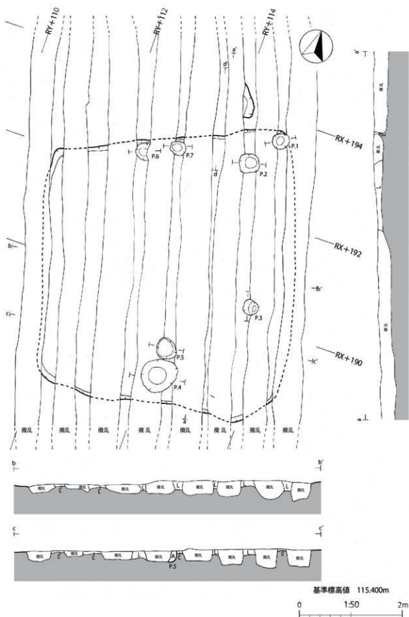
第10圖 RA 059 豎穴建物跡(1)
