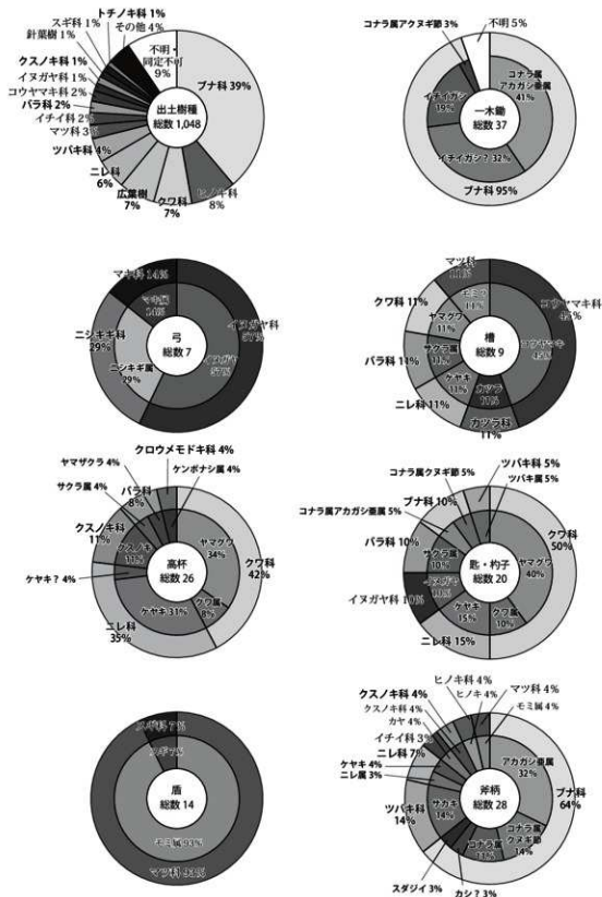
第2図 唐古・鍵遺跡の木製品別にみた樹種選択の傾向
