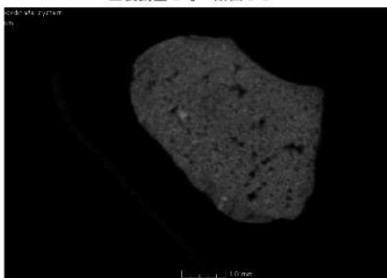
土製鑄型 2号 断面 c-c'
