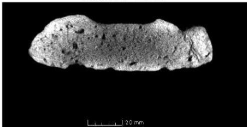
土製鑄型8号 断面 e-e'
