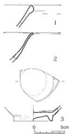
第15図 陶磁器実測図 (1/3)
