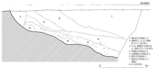
第7図 調査区東側東壁土層断面実測図 (1/40)
