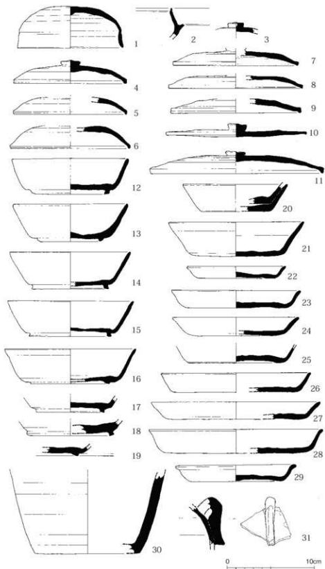
第13図 須恵器実測図① (1/3)
