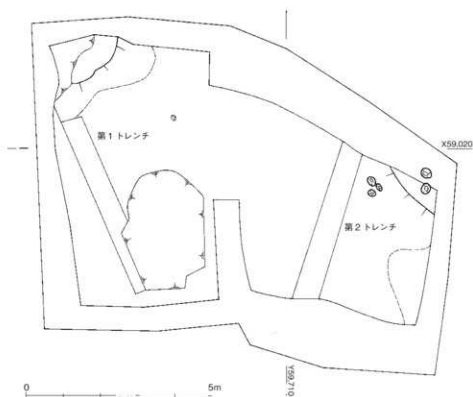
第4図 堂園遺跡1次調査遺構配置図 (1/100)
