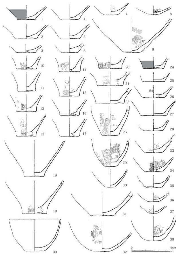
第10图 弥生土器实测图③(1/4)
