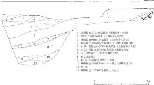
第5図 調査区西側第1トレンチ土層断面実測図(西壁) (1/40)
