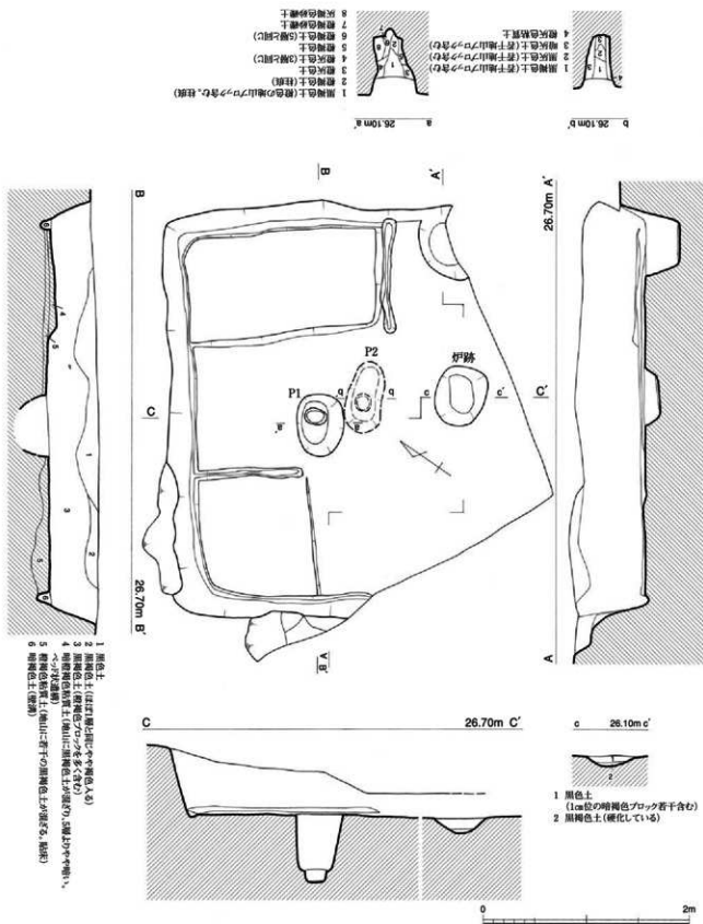
第4図 竪穴住居跡実測図 (1/40)
