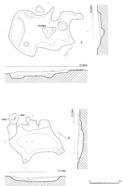
第6图 3·4号土坑实测图(1/30)
