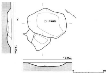
第5図 2号土坑実測図(1/30)
