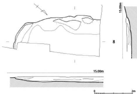
第9図 8号土坑実測図(1/60)
