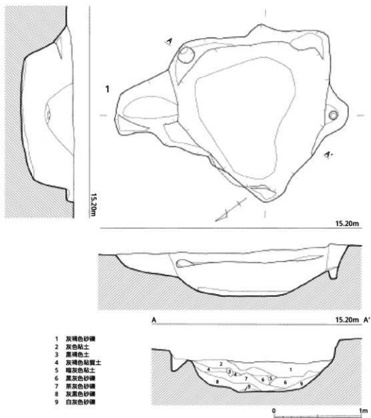
第4図 1号土坑実測図（1/30）
