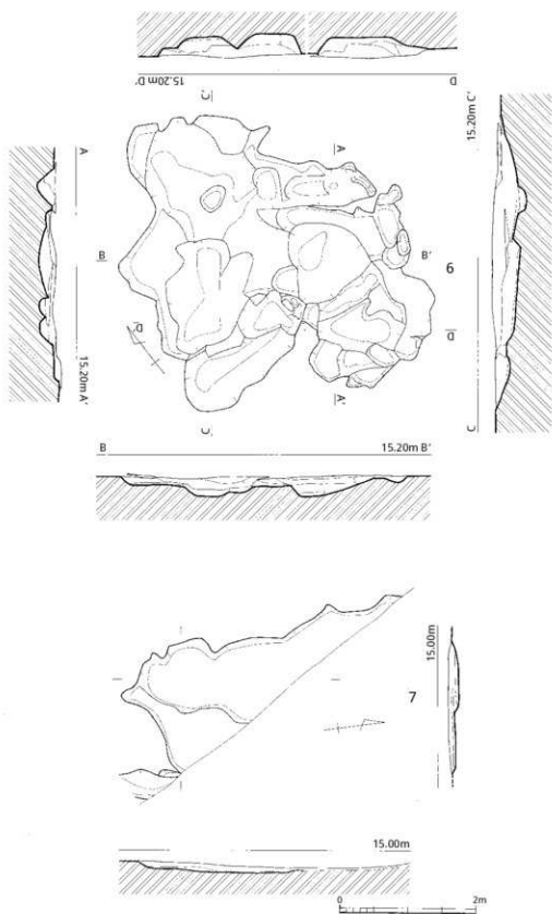
第8图 6·7号土坑实测图(1/60)
