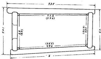
(尺ハ位單ヲ長ノ底下棺石ハ内弧括、ヲ長ノ端上ハ兼計) 圖面平壁棺石 圖三第
