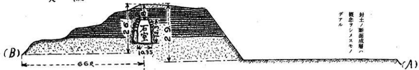
圖面斷(横)線B-A
