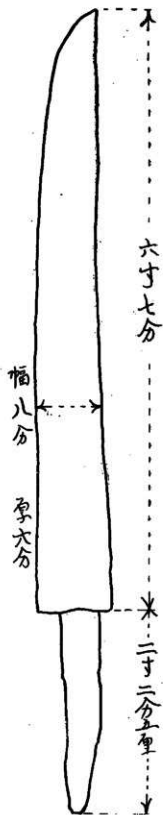
刀子(に号)鞘拓本及寸法
