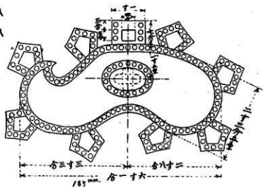
櫛 復原図(い号) 重量 四百七克 櫛板ト銜身ノ取付方 身ノ頭端ヲ之ニ対応スル櫛板ノ穴ニ挿 入シ之ニ鑲嵌(幅二分五厘位)ヲ嵌 入シ、其ノ上ニ槽凹形ノ蓋金物(カバ) ヲ取付ケタリ。
