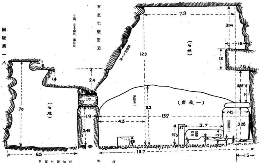
石室北壁面圖
