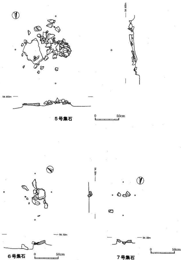
第9図 遺構 (2)
