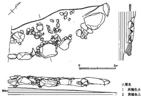
第44図 築石遺構 SX7 実測図 (1/60)
