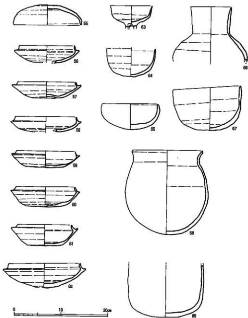
第15图 3号土坑出土遗物实测图 (1/4)
