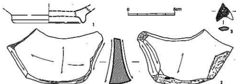
第18図 1号竪穴住居跡出土遺物実測図(1/2)
