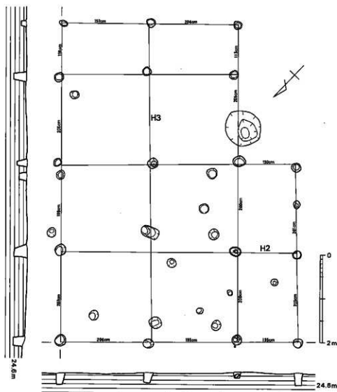
第30図 2・3号掘立柱建物跡実測図(1/60)
