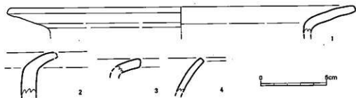
第24図 4号竪穴住居跡出土遺物実測図①(1/2)
