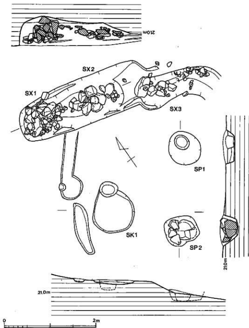
第42図 茶石遺構 SX1～SX3・祠状遺構実測図 (1/40)
