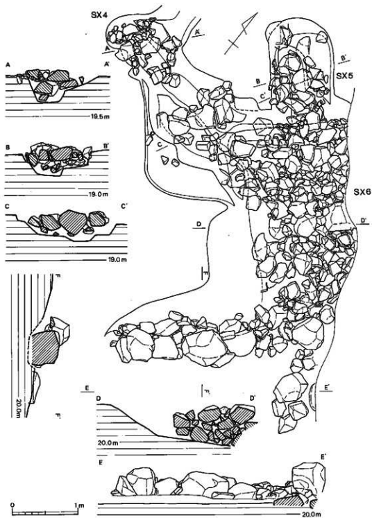
第43圖 集石遺構 SX4 - SX6 実測図 (1/40)
