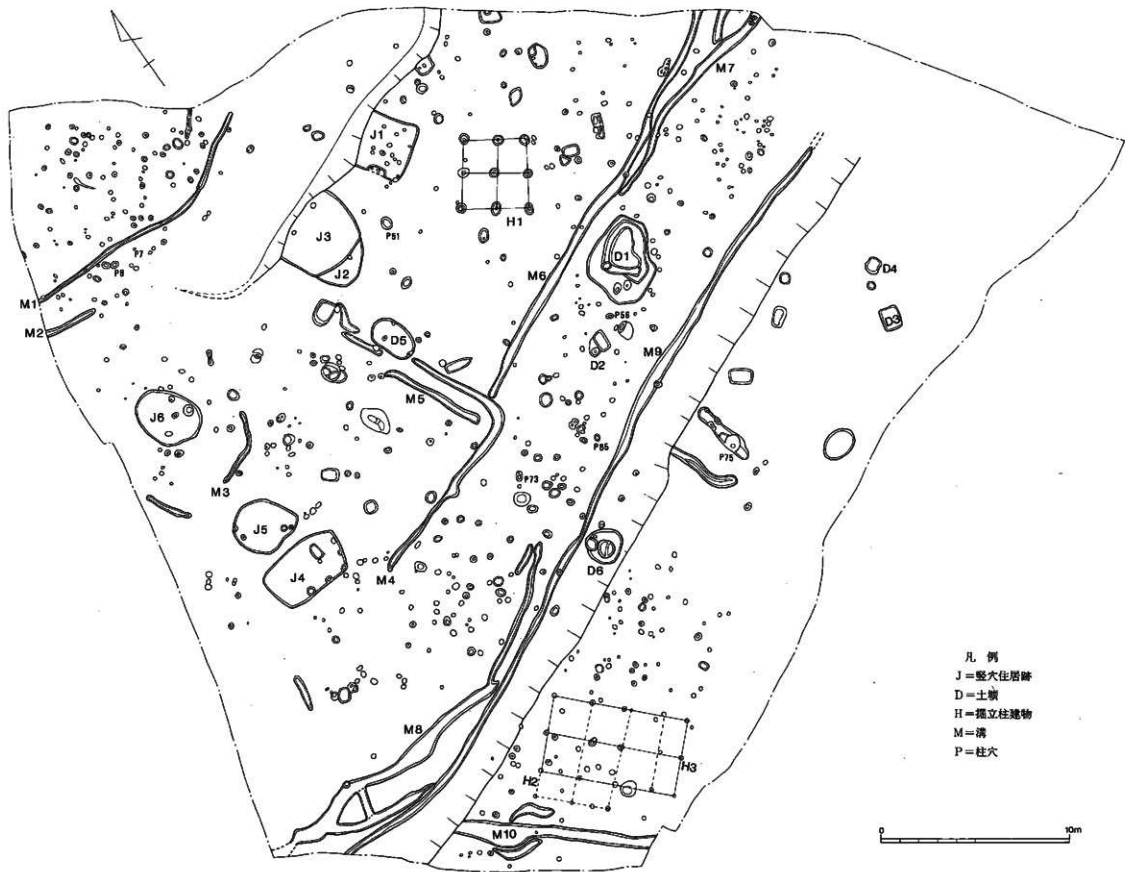
第16圖 田後遺跡第2次調査遺構配置圖(1/200)
