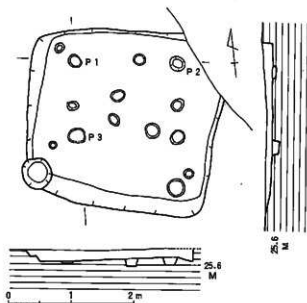
第6図 3号壑穴住居跡実測図 (1/60)
