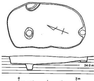
第37図 5号土壙実測図(1/40)
