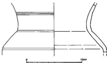
第32图 1号土壕出土器物实测图(1/2)
