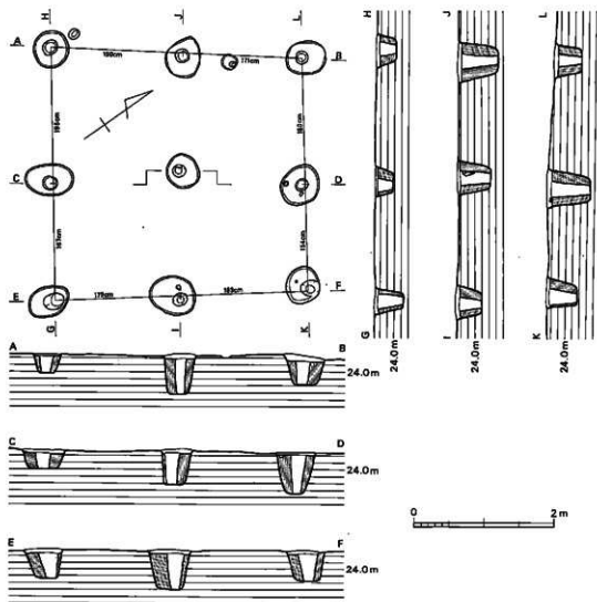
第28図 1号掘立柱建物跡実測図(1/60)
