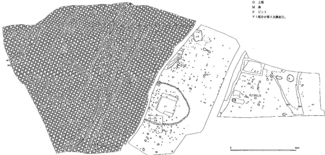
付図2 団後遺跡全体遺構配置図 (1/300)
