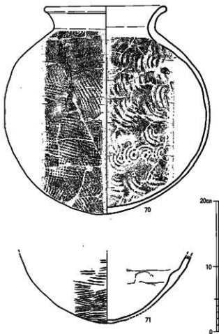
第13図 3号土坑出土遺物実測図 (1/4)
