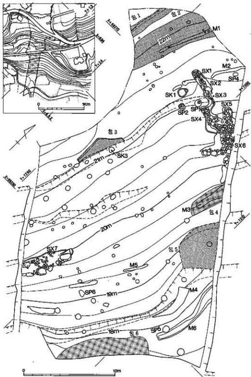
第41圖 遺構配置圖 (1/200)
