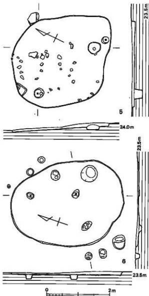
第26図 5・6 竪穴住居跡実測図(1/60)
