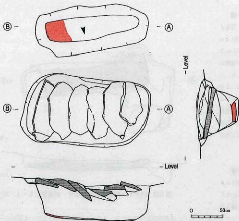
第11図 白木上ノ原遺跡第4号墓平・断面図 (S = 1/30)
