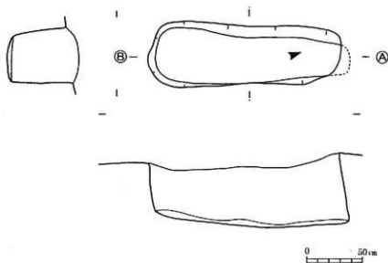
第15図 臼木上ノ原遺跡第8号墓平・断面図 (S = 1/30)
