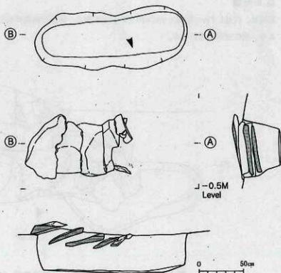
第12図 白木上ノ原遺跡第5号墓平・断面図 (S = 1/30)
