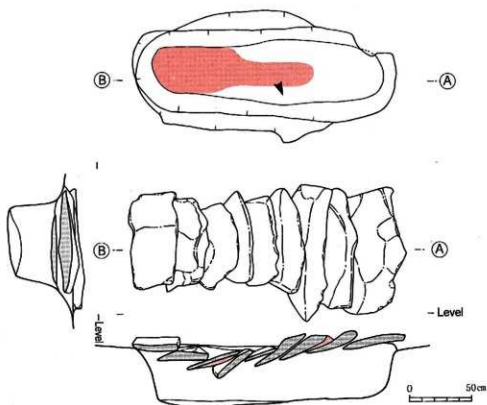
第9図 白木上ノ原遺跡第2号基平・断面図 (S=1/30)
