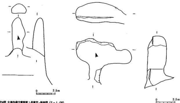
第34図 大源寺横穴墓群第1号墓平・断面図 (S=1/60)
