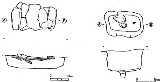
第17図 臼木上ノ原遺跡第10号墓平・断面図 (S=1/30)
