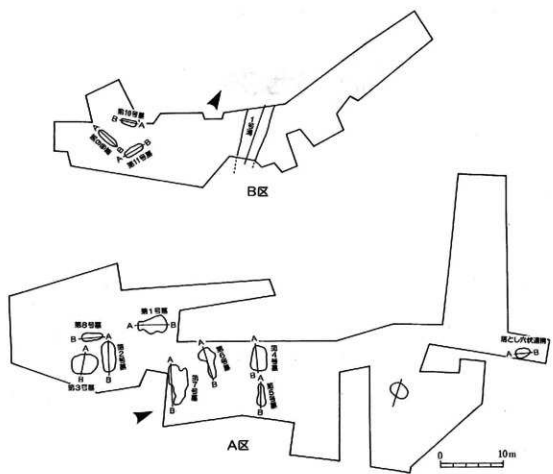
第7图 白木上ノ原遺跡遺構配置図 (S=1/300)
