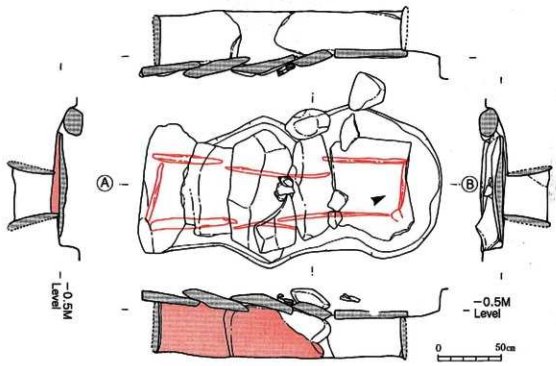
第8图 白木上ノ原遺跡第1号墓平・断面図 (S=1/30)
