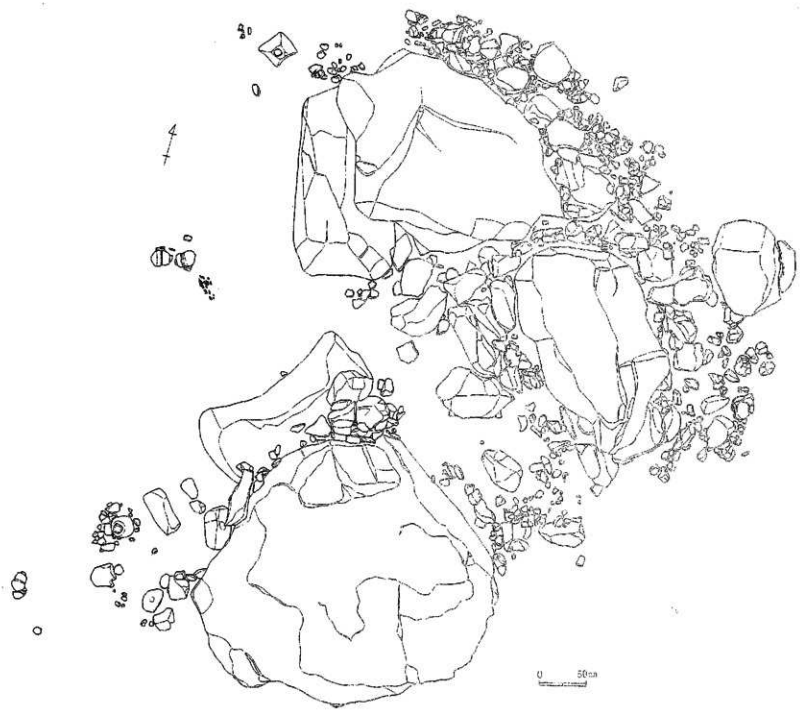
第4圖 瑞雲遺跡平面圖 (S=1/40)
