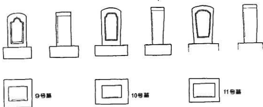
第7图 近世墓 正·侧面图(1) (1/20)
