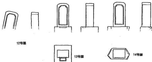
第8図 近世基 正・側面図②(1/20)
