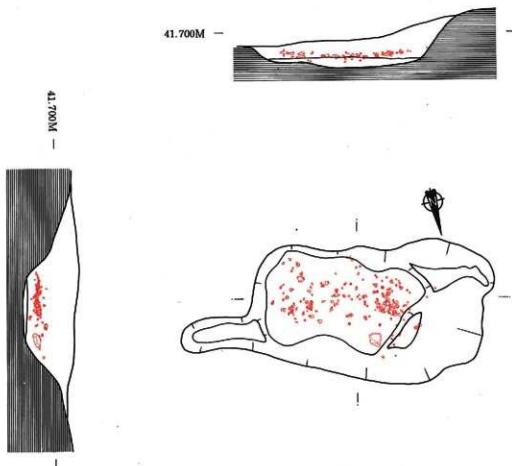
第3図 SK1 平・断面図(1/100)
