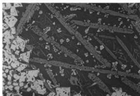
写真 31 顕微鏡写真 (資料 NO. 1-2) × 100
