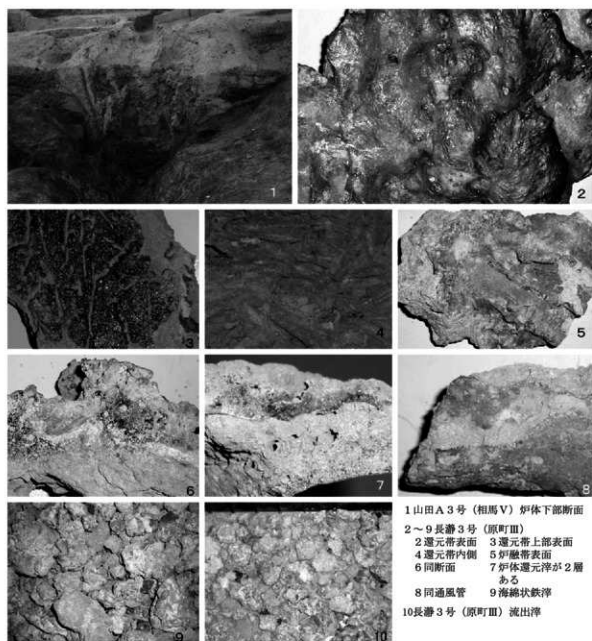
図11 筒形製鉄炉関連資料
