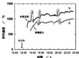
図3 操作時の炉内温度の推移
