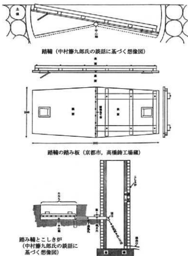
図6 参考にした踏み輪
