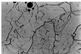
写真 53 鉄組織写真 (資料 NO. 2) \times 100
