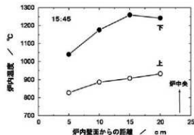
図5 15:45における炉内温度分布
