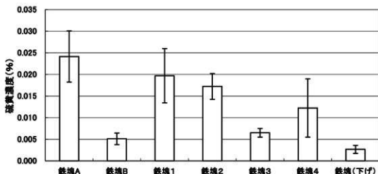
図4 鉄塊試料中の硫黄濃度
