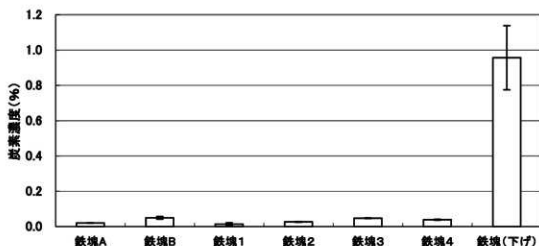
図3 鉄塊試料中の炭素濃度
