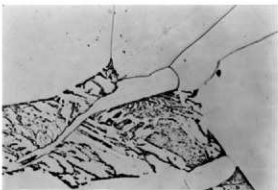
写真 62 鉄組織写真 (資料 NO. 7-2) × 400
