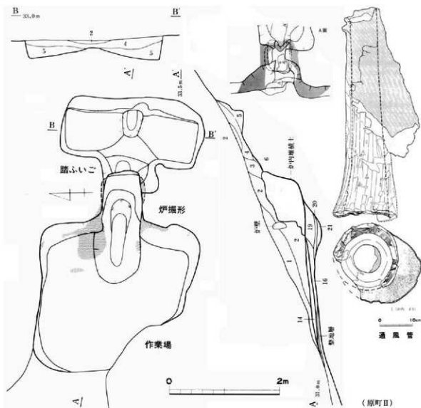
図10 長瀨3号製鉄炉跡
