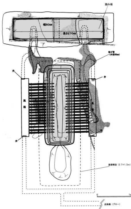
図8 まほろん2号炉と15号製鉄炉
