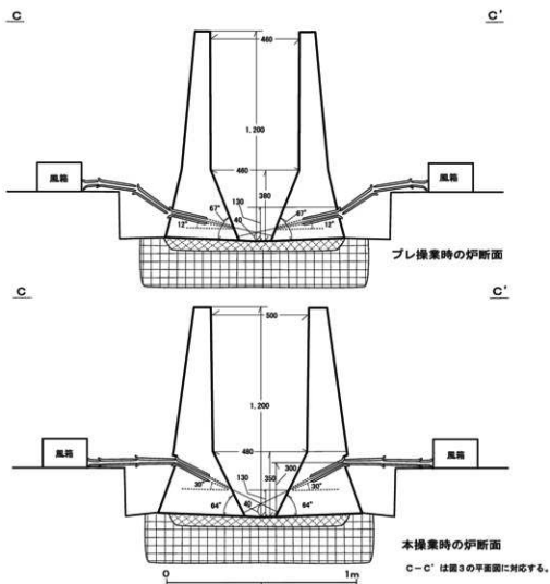
図15 まほろん2号炉の断面（構築時）
