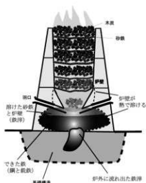
図17 一般に考えられる炉内状況
