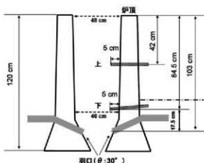
図1 炉の断面図と熱電対の設置位置
