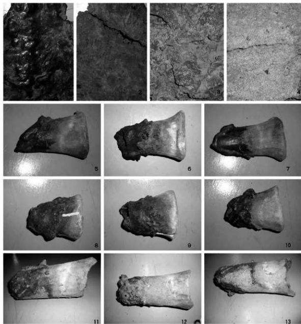
鳥井沢B1号 1 炉体付着還元滓 2 同裏側 3 熔融滓表面 4 同裏側 長瀬6号 5、8、11 羽口側面 6、9、12 羽口上面 7、10、12 羽口下面 (原町III)
