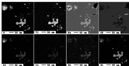
図12 鉄塊（下げ）のEPMA画像
