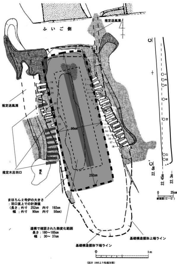
図14 まほろん2号炉の炉壁厚と15号製鉄炉
