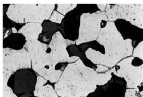
写真 52 鉄組織写真 (資料 NO. 1) \times 400
