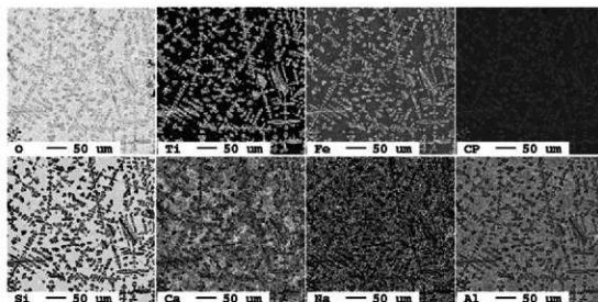
図10 スラグ4BのEPMA解析像
