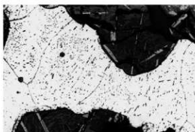
写真 55 鉄組織写真 (資料 NO. 3-1) \times 100
