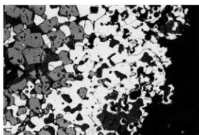
写真 51 鉄組織写真 (資料 NO. 1) \times 100
