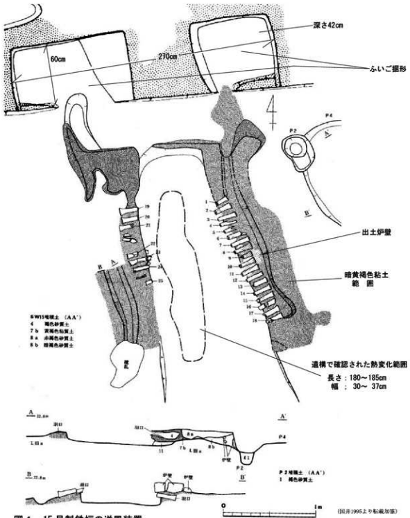
図4 15号製鉄炉の送風装置
