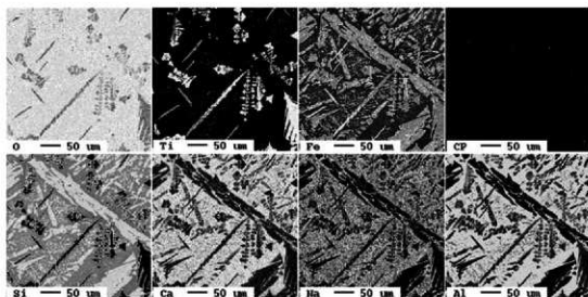
図7 鉄塊1のEPMA解析像
