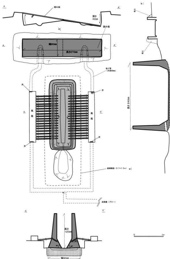
図3 まほろん2号炉
