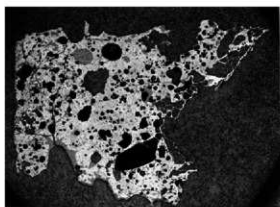
写真 26 マクロ写真 (NO. 1) × 5
