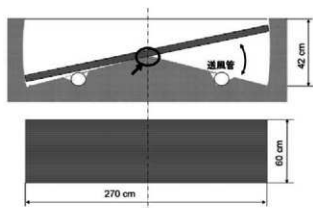
図9 踏み輻の概略図
