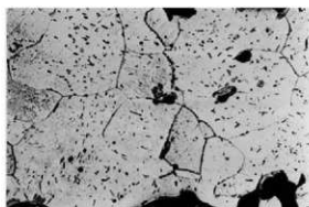
写真 57 鉄組織写真 (資料 NO. 3-2) \times 100
