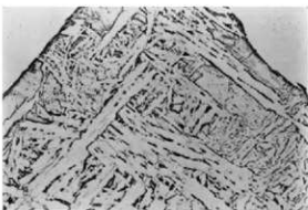
写真 60 鉄組織写真 (資料 NO. 7-1) × 400
