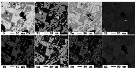
図13 鍛冶滓のEPMA画像
