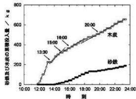
図4 砂鉄と木炭の累積投入量
