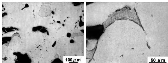
写真8 No. 2位置の粗大な粒状鉄のマイクロ組織
