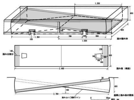
図5 まほろん2号炉の踏みふいご設計図
