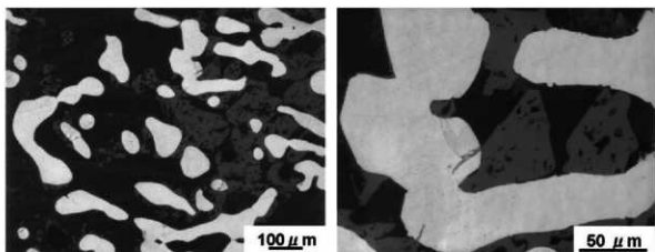
写真6 No. 1位置の小さな粒状鉄のマイクロ組織
