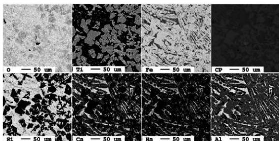
図9 スラグ1のEPMA解析像
