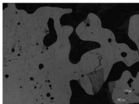
(a) 鉄塊1 金属部分
