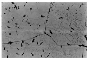
写真 58 鉄組織写真 (資料 NO. 3-2) \times 400
