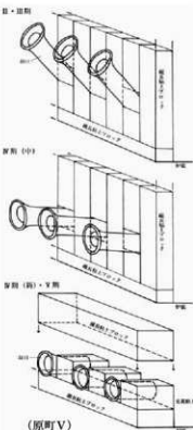
図6 小暮伸之による羽口装着案
