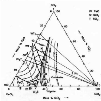
FeO n -SiO 2 -TiO 2 系平衡状態図
