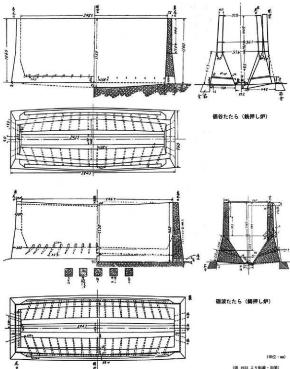
図16 備谷たたらと碓波たたら実測図
