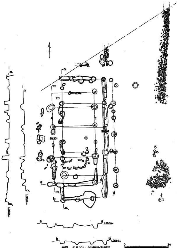
48图 SB201·202建物实测图
