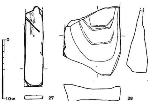
103図 紙石実測図
