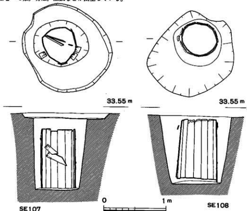
8図 SE107・108井戸実測図
