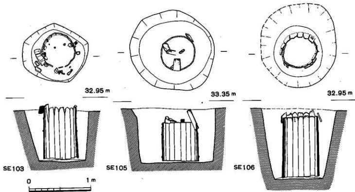
7图 SE103・105・106井戸実測図
