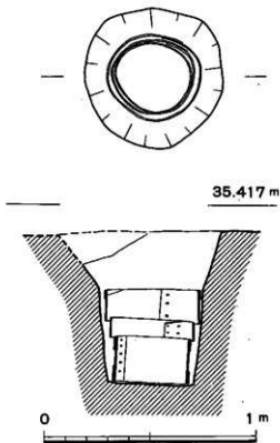
49図 SE206井戸実測図
