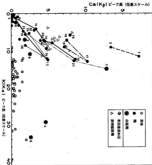
135図 陶磁器破片(太宰府町御笠川南条坊遺跡出土)の茶地及び軸についてのカルシウム(K \beta 線)蛍光X線強度とカリウム(K \alpha 線)蛍光X線強度との相関 ここに参照のために西有田町原明古窯跡出土の磁器軸についての対応するプロットとともに、有田周辺の陶磁器原料石についての対応するプロットも示した。
