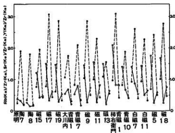
132図 有田周辺古窯跡出土の陶磁器破片についての重金属成分（ルビジウム、ストロンチウム、イットリウム）のジルコニウムに対する蛍光X線強度比プロット
