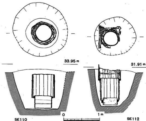
5図 SE110・112井戸実測図
