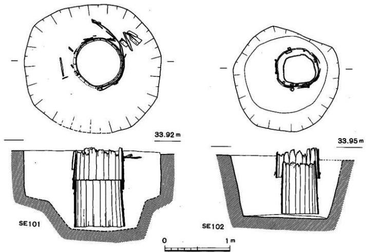
6图 SE101・102井戸実測図
