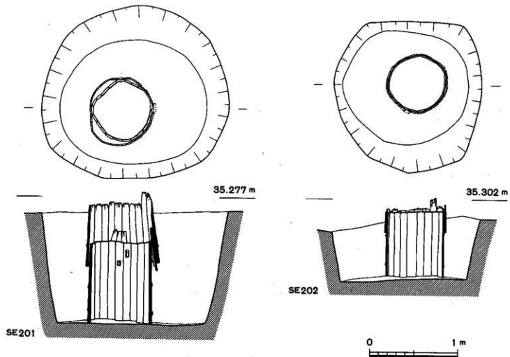
51图 S E 201 · 202井戸実測図
