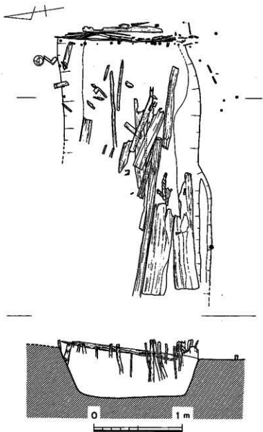
9圖 S X101不明遺構実測図
