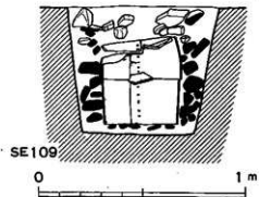
4図 SE109井戸実測図
