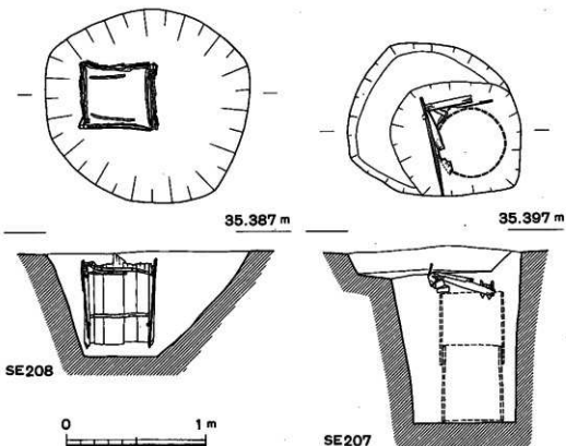
50図 S E.207・208井戸実測図
