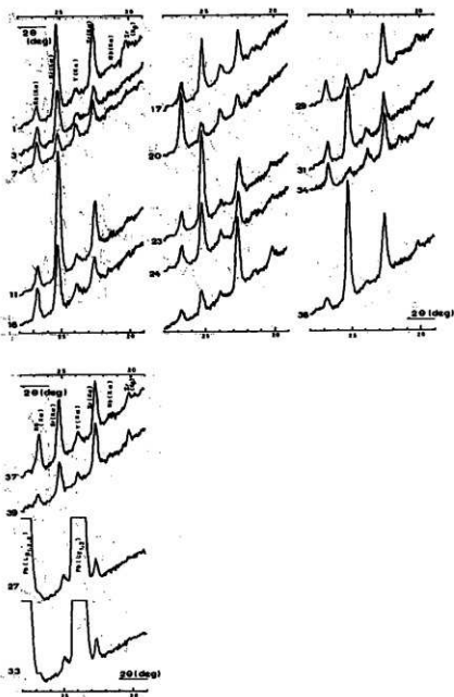
128図 陶磁器破片の釉についての重金属成分( 2\theta=19^\circ\sim 28^\circ 域)の蛍光X線スペクトル (試料番号は33表に準ずる)
