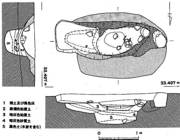
54図 SX201窯跡実測図
