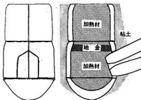
120図 銅地金溶解方法想定模式図
