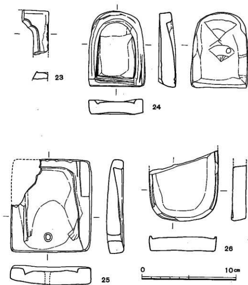
102図 石製硯実測図
