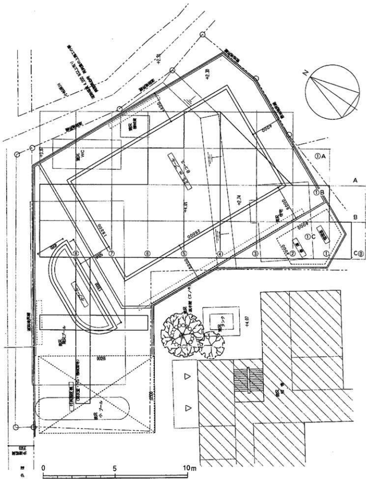
第3図 本渡北小学校プール造替調査区域図
