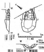
図8 SK01平・断面図
