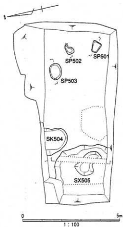
図4 第5層下面検出遺構平面図(1:100)
