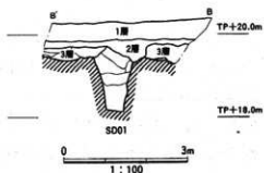
図3 基本層序とSD01断面図
