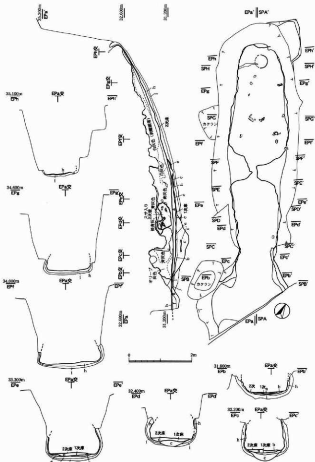
第41図 9号窯 平面図・断面図・左側壁図 (S=1/60)
