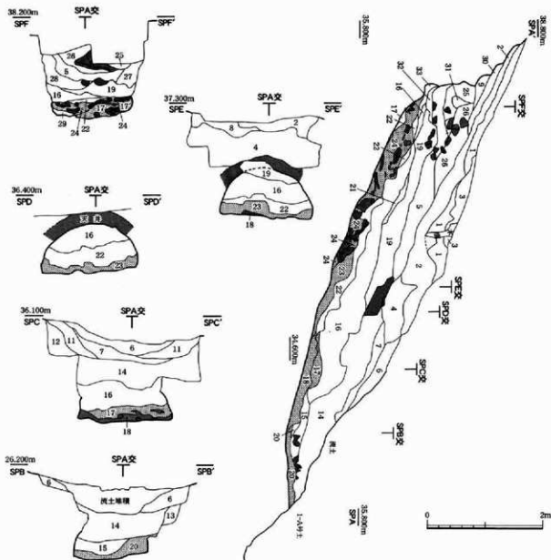
第9図 2号塚 埋土セクション図 (S=1/60)
