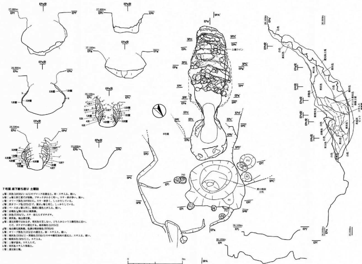
第29図 7号窯 平面図・断面図 (S=1/40)
