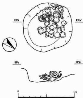
第21図 A地区 SK4平面図・断面図 (S=1/20)
