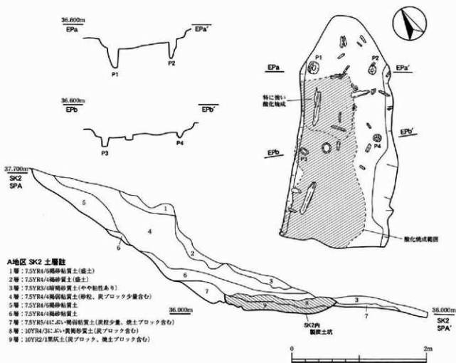
第18図 A地区 SK2セクション図、SK2内製炭土坑平面図・ビットエレベーション図 (S=1/40)
