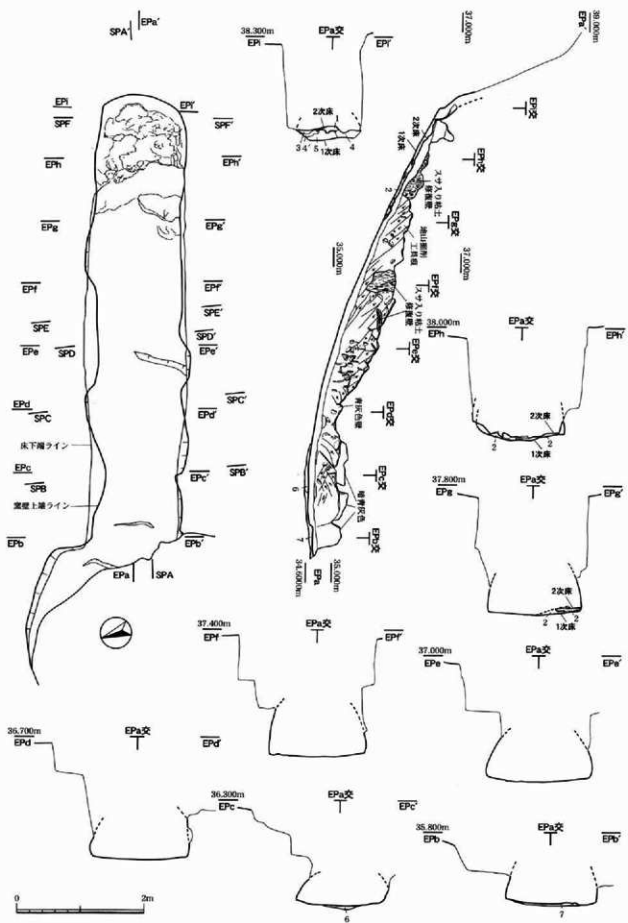
第7図 2号窯平面図・断面図 (S=1/60)
