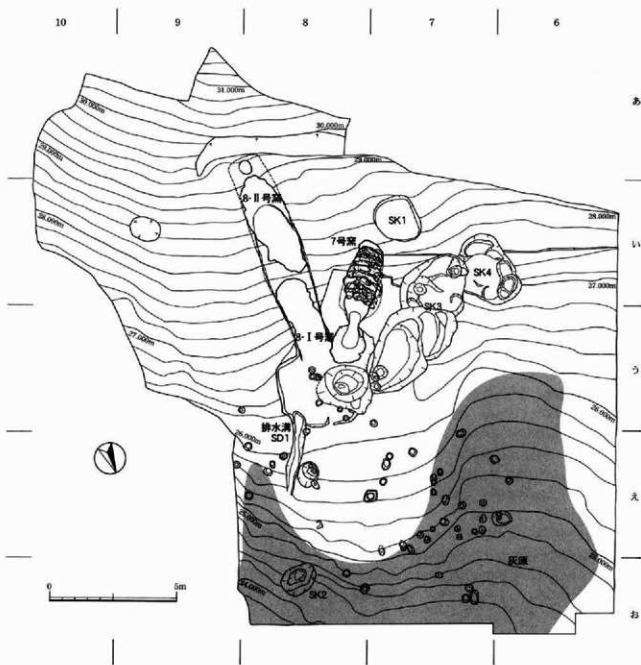
第23図 B地区 遺構検出地区全体図 (B地区南東側1/2区域) (S=1/150)
