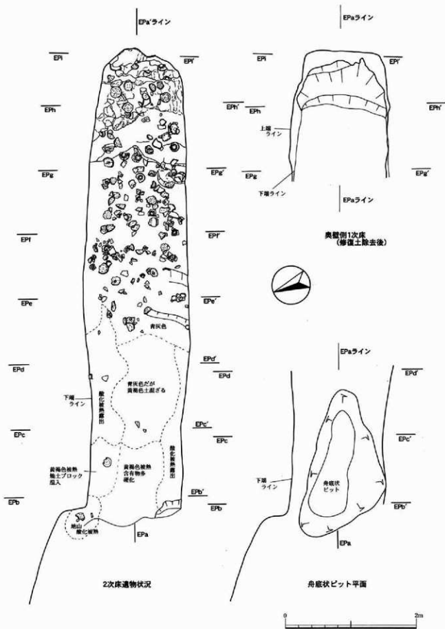
第8図 2号竊床面遺物出土状況図 (S=1/40)
