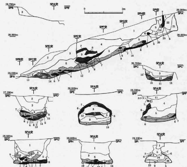
第27図 8号煤 埋土セクション図 (S=1/60)
