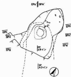
第42図 9号窯 後背部テラス平面図 (S=1/60)
