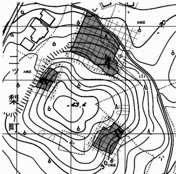
第5図 本調査区グリッド配置図 (S=1/1,000)
