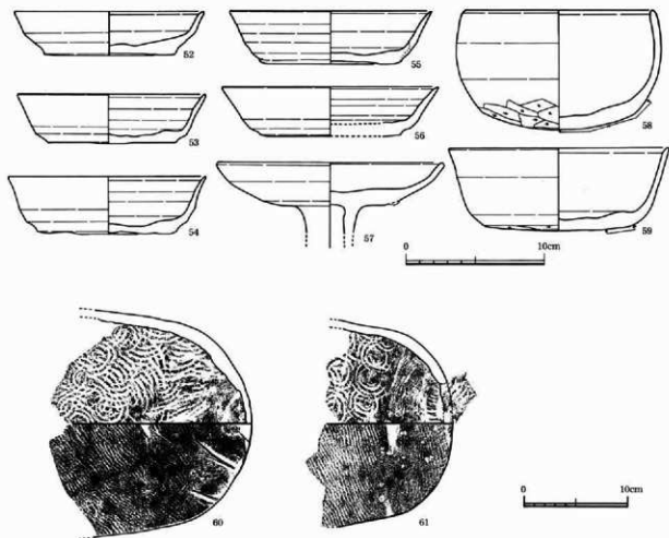
第49図 2号窯 床出土 須恵器(3) (S=1/3)
