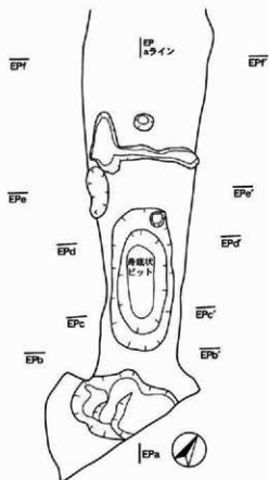
第43図 9号窯 床下遺構平面図 (S=1/60)
