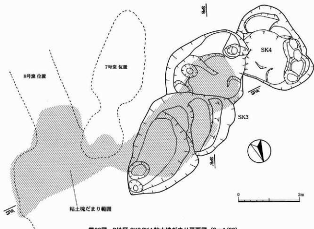
第33図 B地区 SK3,SK4,粘土塊だまり平面図 (S=1/60)
