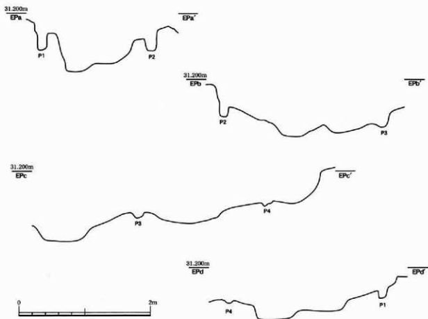
第20図 A地区 SK5ビットエレベーション図 (S=1/40)
