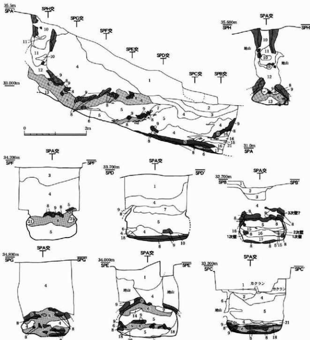
第46図 10号窯埋土セクション図 (S=1/60)
