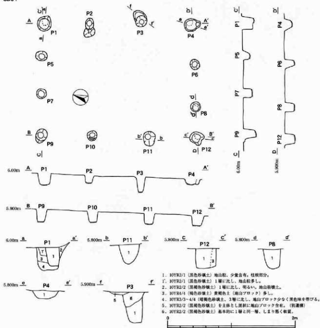
第4図 SB01 平面及び断面図 (平面・エレベ図・S=1/60, 土層断面図・S=1/30)
