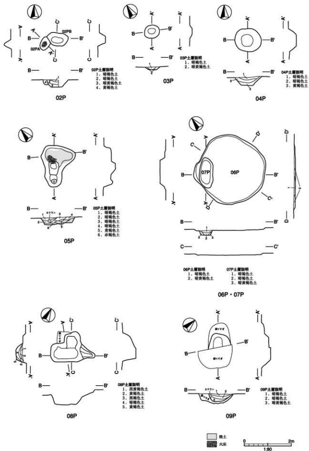
第25図 二重堀遺跡 e 地点炉穴・土坑実測図
