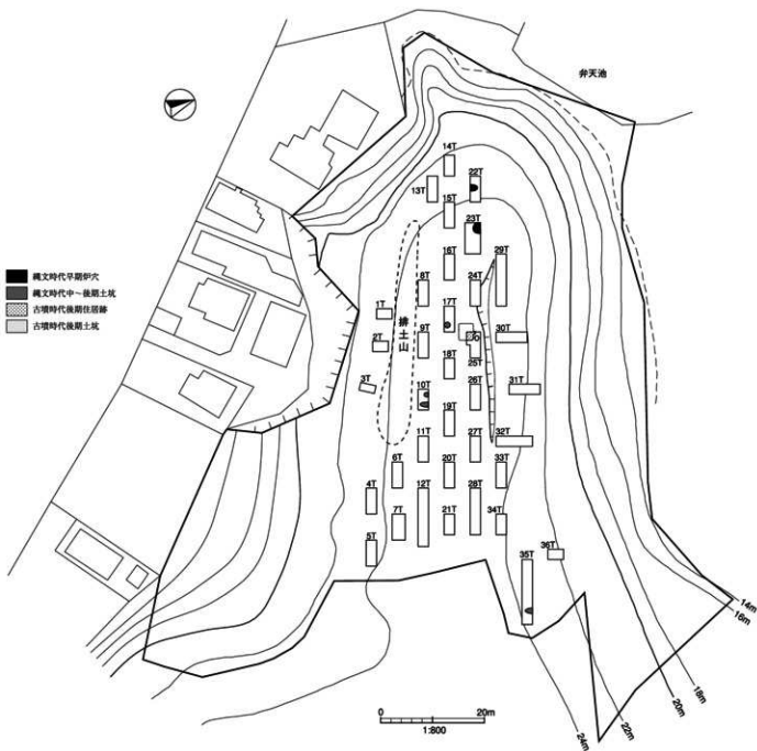
第31図 本郷台遺跡遺構検出状況図
