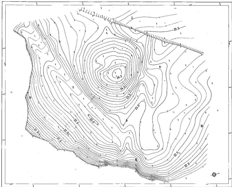
第5図 菅地ノ台古墳測量圖 (1 : 200)
